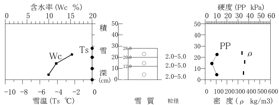
積雪断面観測値（構内 2024/12/25）
