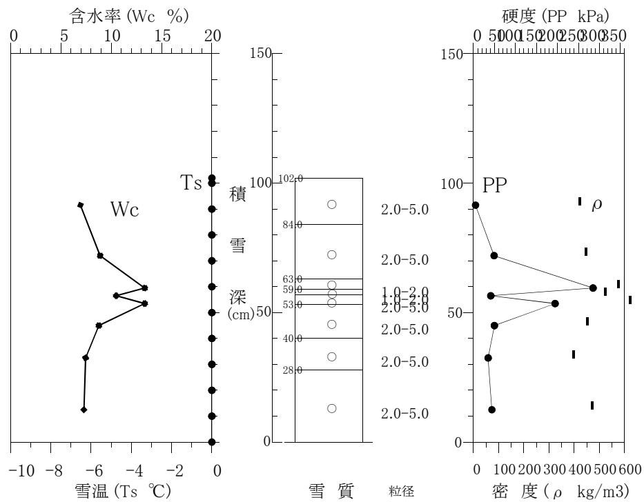
積雪断面観測値 (構内 2025/03/14)
