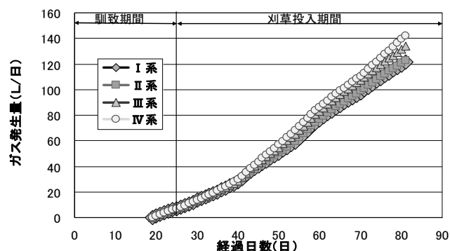
図-2.2.1-13 I～IV系の累積ガス発生量の推移
