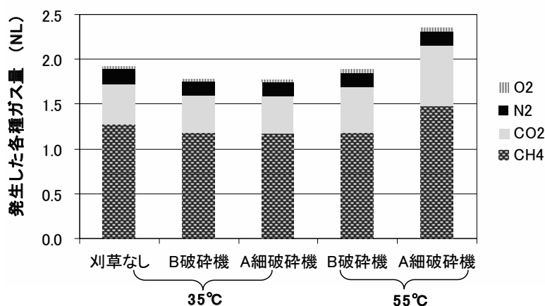
図-2.2.3-1 各条件による汚泥及び刈草の消化ガス発生量
