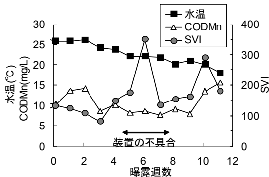
図-5.5 h-AS 処理水と汚泥性状
