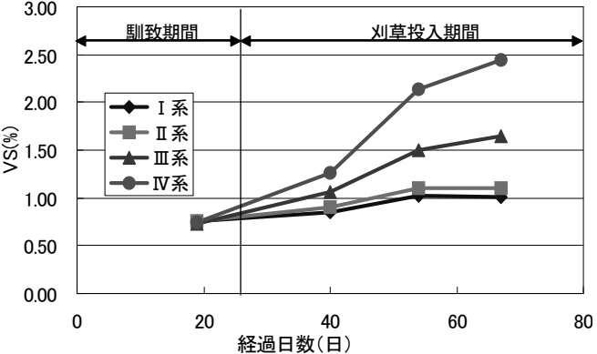
図-2.2.1-5 I～IV系の VS の推移
