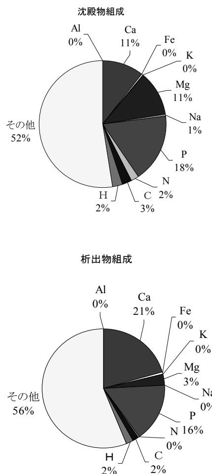
図 3.8 消化汚泥脱水分離液を電解したときの回収物組成
