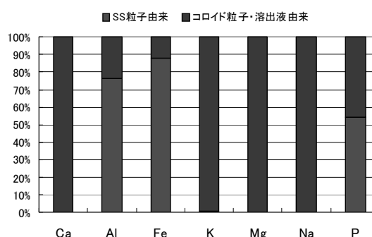
図 4.10 各元素の流出量の構成 (No.4)
