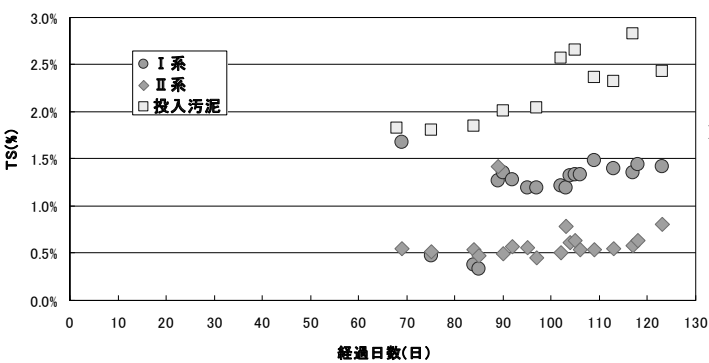
図-2.3.3-2 各条件における引抜汚泥の TS の推移
