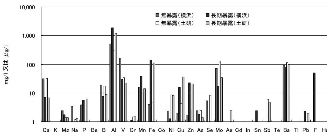
図 3. 3. 3 環告 46 号試験における各元素の溶出挙動
