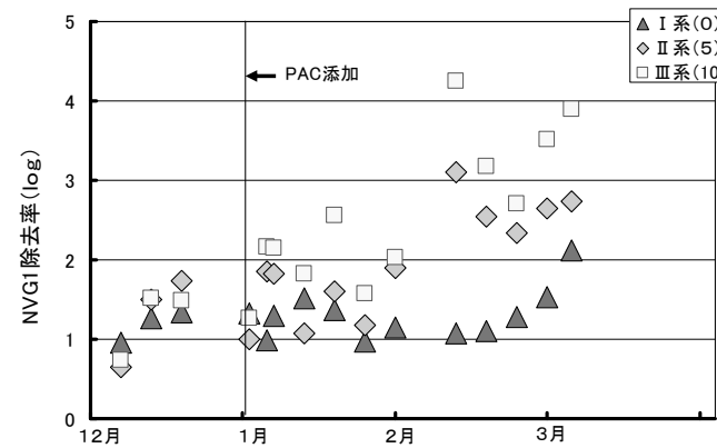
図-4 凝集剤添加による除去率の推移(G1)
