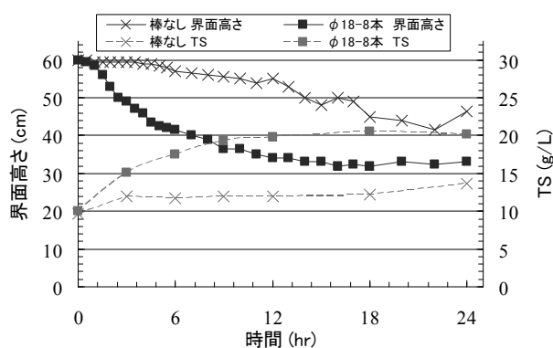
図 2.8 沈降曲線と底部濃度（初期汚泥濃度 10g/L）
