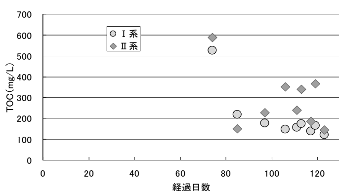
図-2.3.3-8 各条件における TOC の推移
