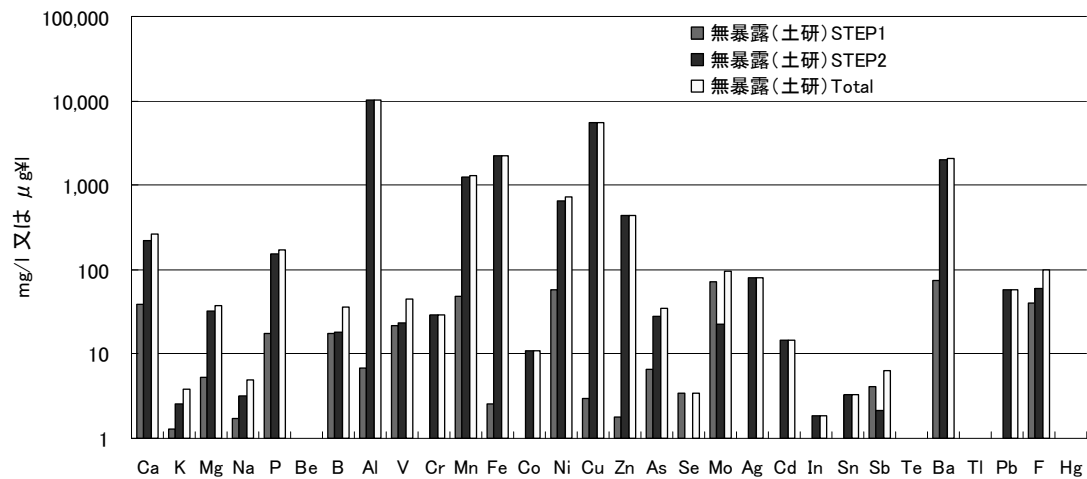
図3. 3. 6 最大溶出可能量試験（酸系列・土研試料）における各元素の溶出挙動 (Be,Te,Tl,Hg については定量下限値未満) (単位は、Ca,K,Mg,Na,P については mg/l、その他については \mu g/l)
