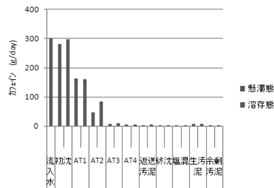
図-3.15 カフェインのフラックス
