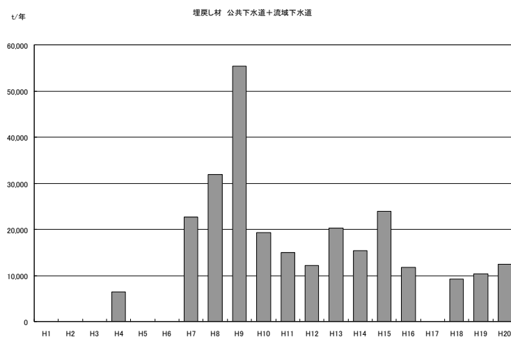
図4. 2. 6 埋戻し材製造量の経年変化
