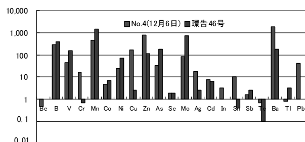
図 4.11 環告 46 号試験との比較 (Al, Fe など土壤からの流出量が非常に大きく、環告 46 号の試験結果を上回っている元素は除く)
