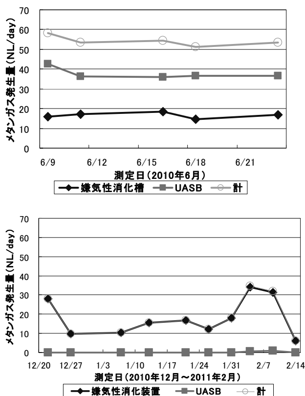
図 3.3-5 UASB-AD-AS システムのメタンガス発生量
