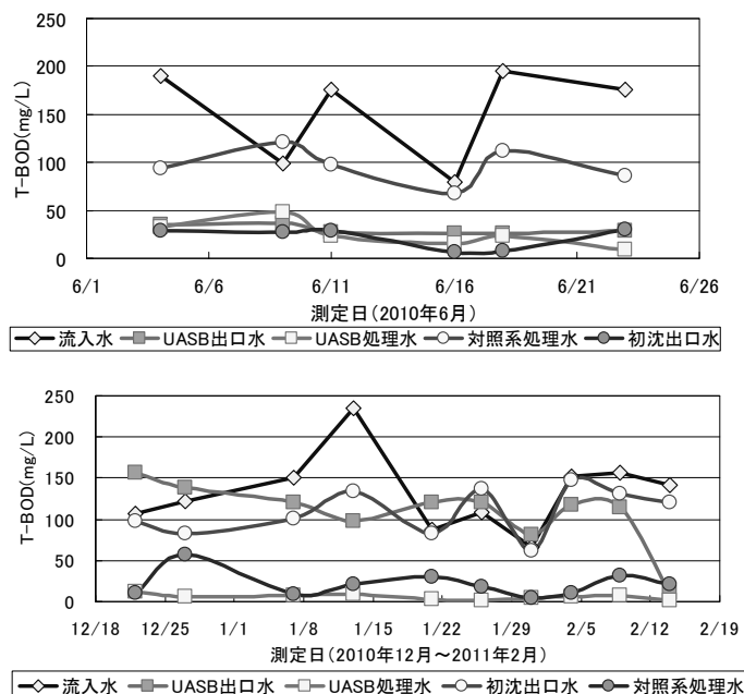
図 3.3-4 UASB-AD-AS システムの T-BOD 処理特性
