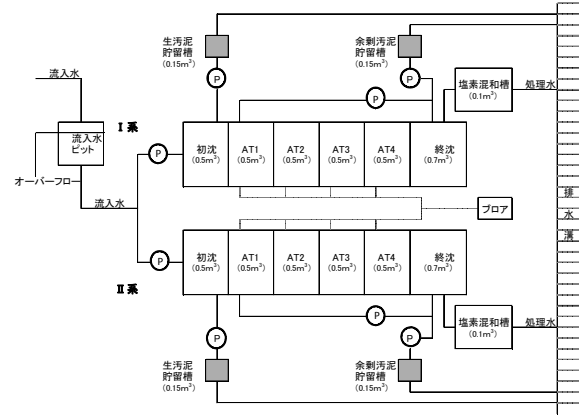
図-3.4 実験装置（概要）
