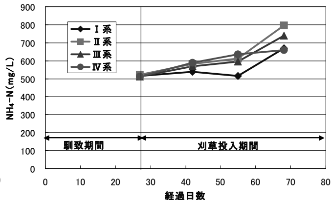
図-2.2.1-12 I～IV系の \text{NH}_4\text{-N} の推移
