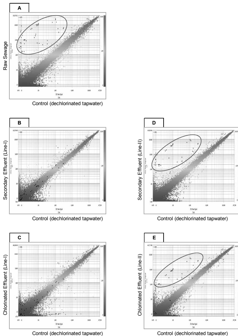
図3.6 脱塩素水道水と各ばく露区の雄メダカ肝臓中の遺伝子発現強度の関係
