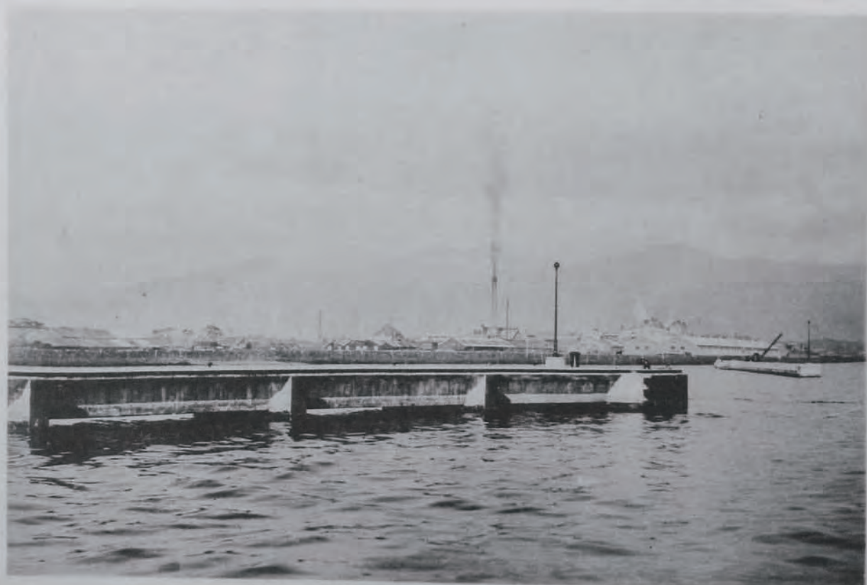
(13) 清水港修築工事 繫船杭及棧橋表側並防波堤
