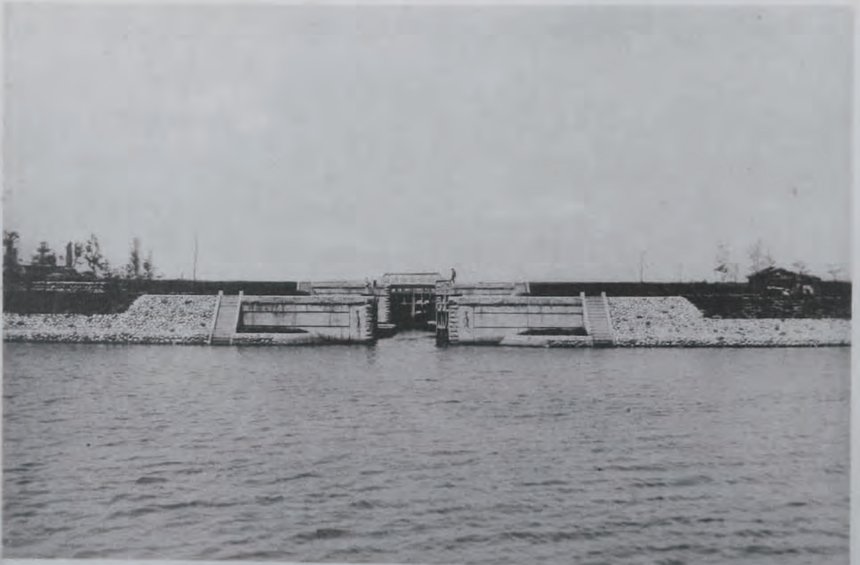
(5) 神通川改修工事萩之浦閘門工事竣功狀況 (富山縣婦負郡草島村地先)
