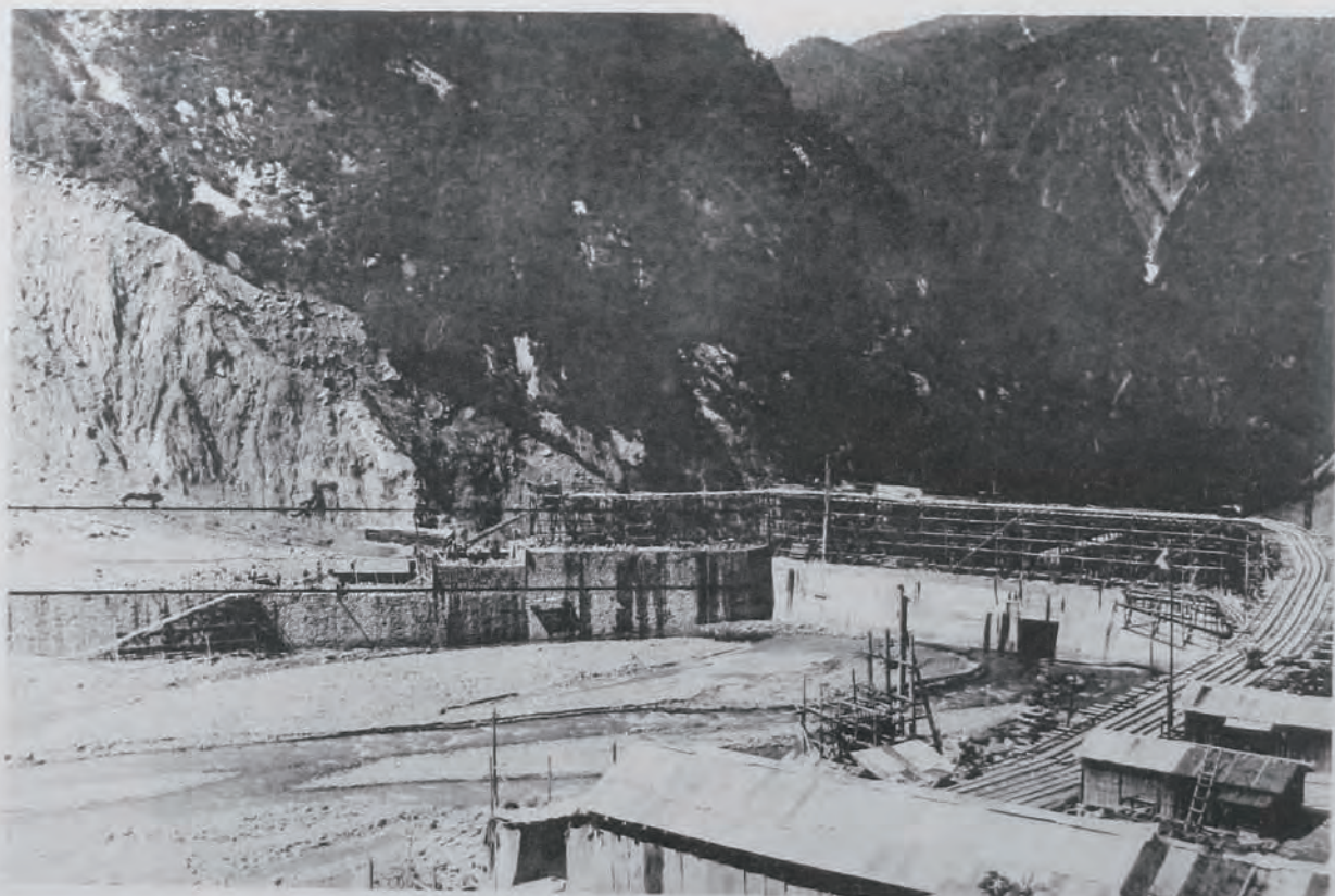
(11) 常願寺川砂防白岩堰堤築設 (右岸上流ヨリ望ム) 第四號護岸下半部施工進行中ノ狀況
