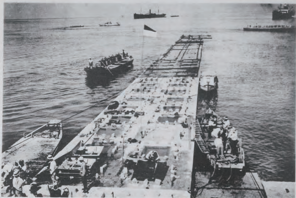
(16) 土崎港修築工事中ノ函塊突堤
