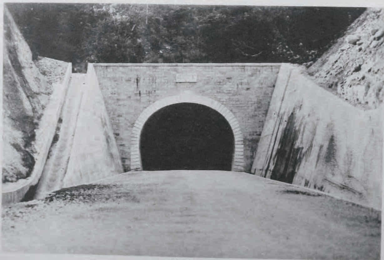
(31) 國道五號線(福島)竣成後ノ栗子隧道 (福島縣信夫郡中野村ヨリ山形縣南置賜郡萬世村大字梓山ニ至ル工事) 福島口ヲ望ム
