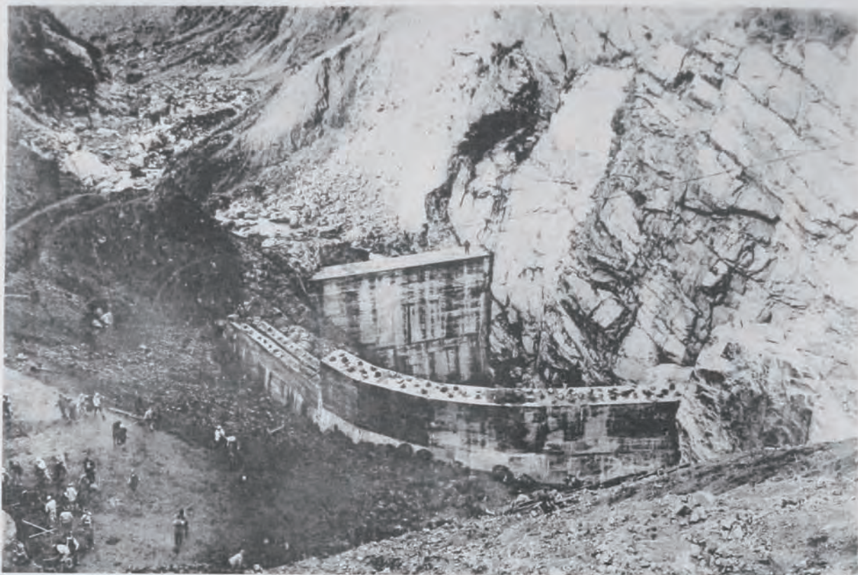
(10) 常願寺川砂防白岩堰堤築設 (下流高所ヨリ望ム) 裏埋土留擁壁竣功ノ狀況
