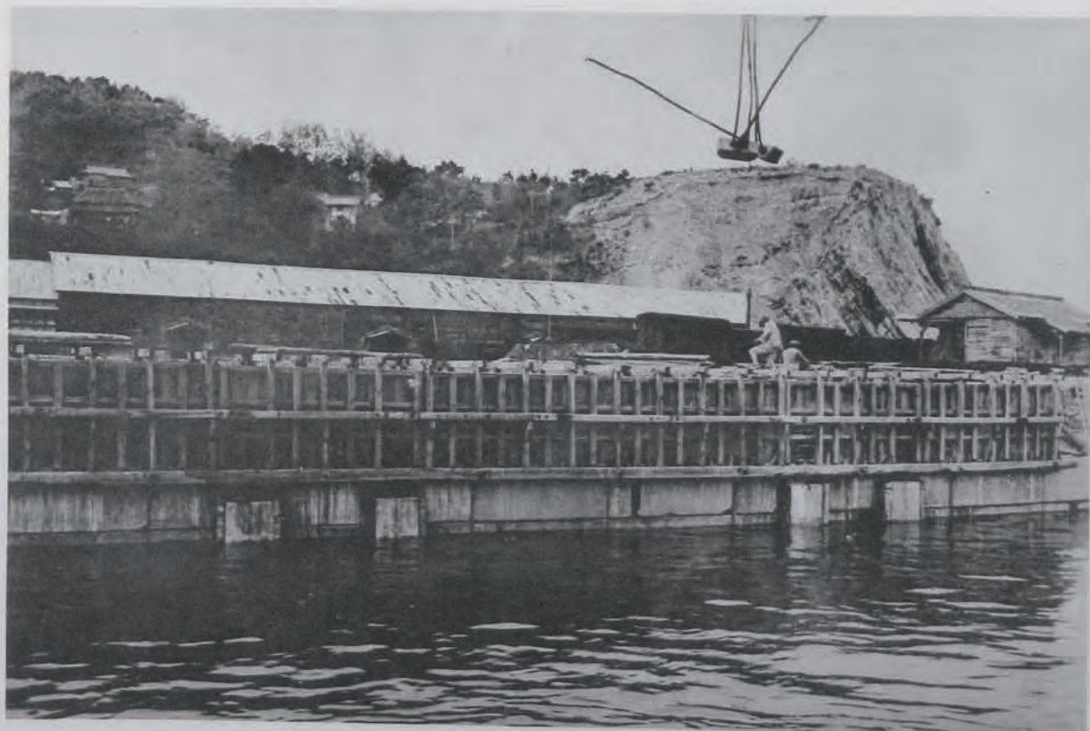
(19) 三角港修築工事岸壁 八米岸壁A部頂部混凝土型枠組立
