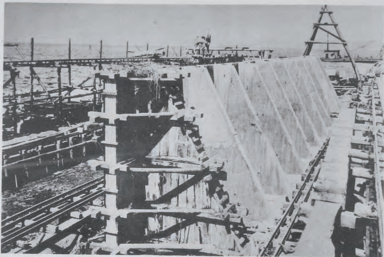
(18) 青森港修築工事物揚場護岸 扶壁付L形塊製作、塊ノ高四米四、幅二米、重量約十五噸
