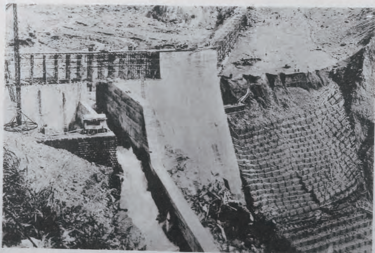
(9) 常願寺川砂防白岩堰堤築設(下流ヨリ望ム) 護岸裏埋法面被覆工木工沈床滑落ノ状況
