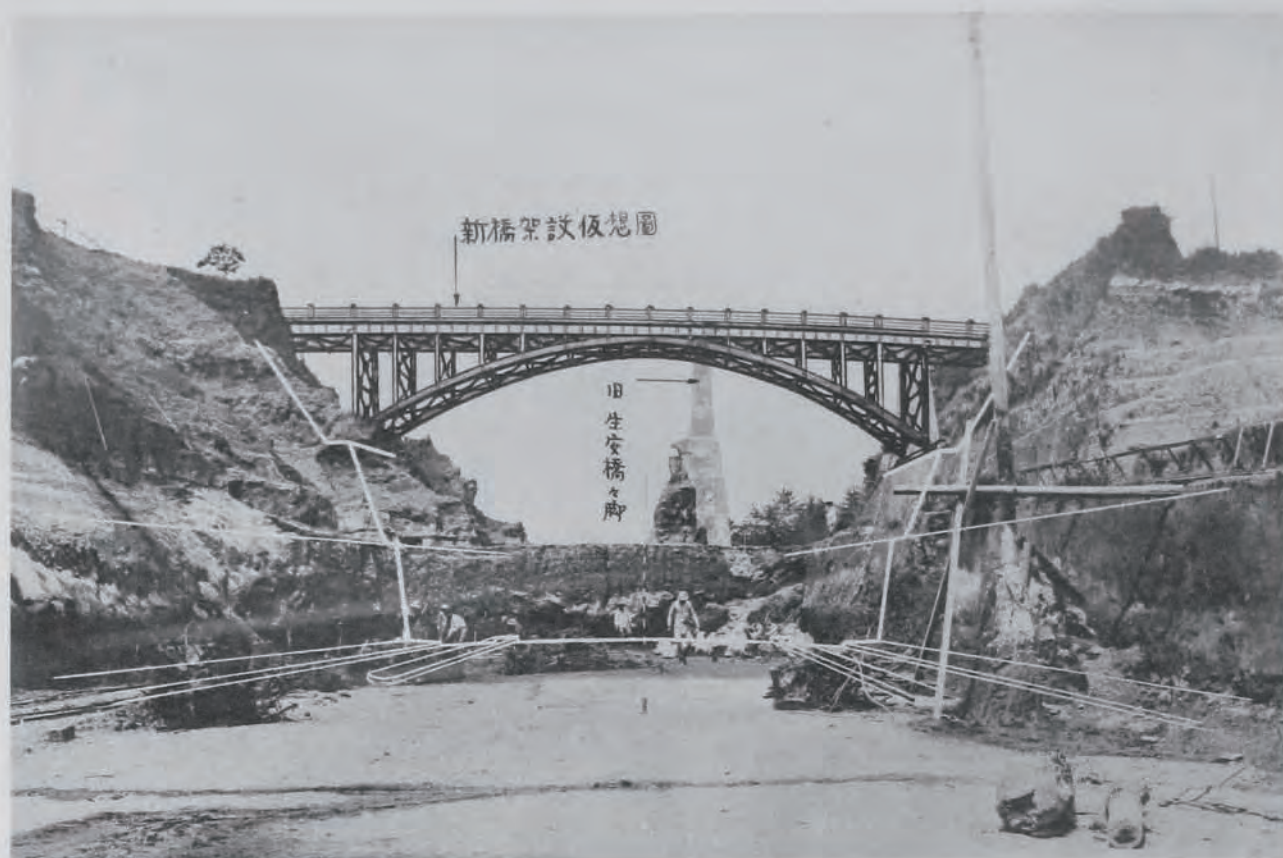
(29) 國道一號線改良工事計畫 測點三百九十號ヨリ三百八十六號ヲ望ム (横濱市鶴見區生麥町地内)
