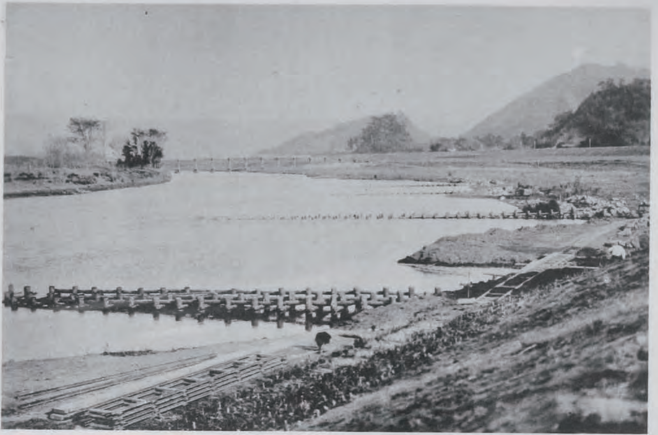
(15) 狩野川改修工事大平水制 杭出七列、延長百五十七米 (静岡縣駿東郡大平村地先)
