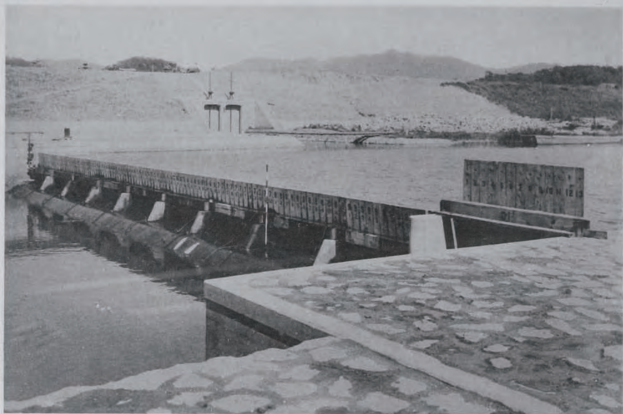
(7) 圓山川改修附帶工事新田用水堰
