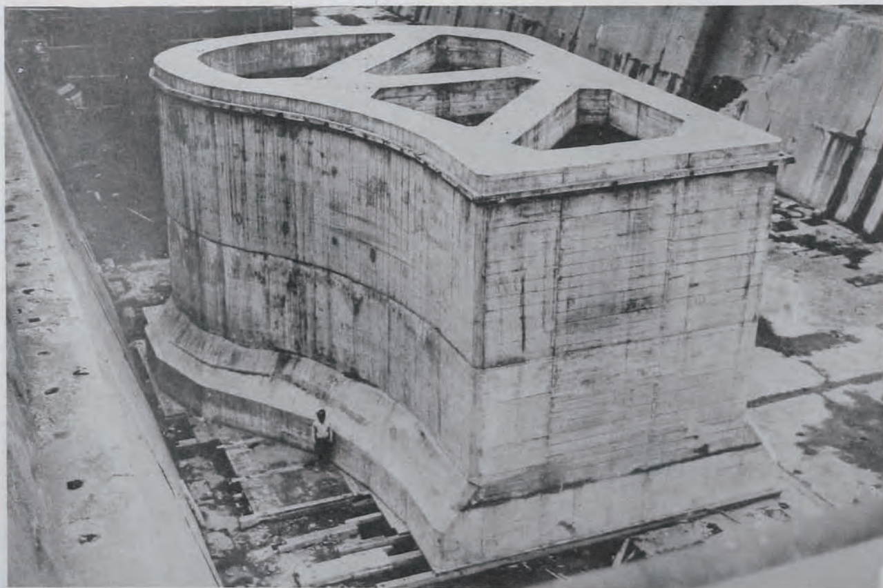
(24) 横濱港修築工事外防波堤副堤頭南
