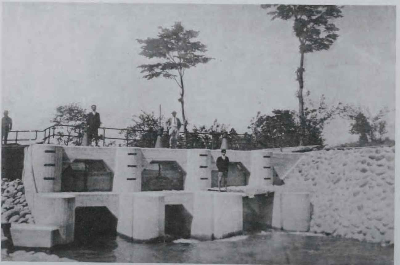
(6) 神通川改修附帶工事通水狀況 用水路改築第一號水門 (富山縣上新川郡大久保町大字鹽、神通地先)
