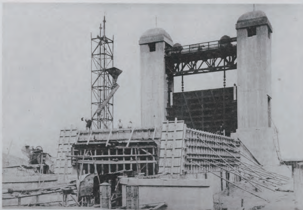
(10) 紀ノ川改修工事水軒川水門 スラブ型枠組立及混凝土作業ノ状況
