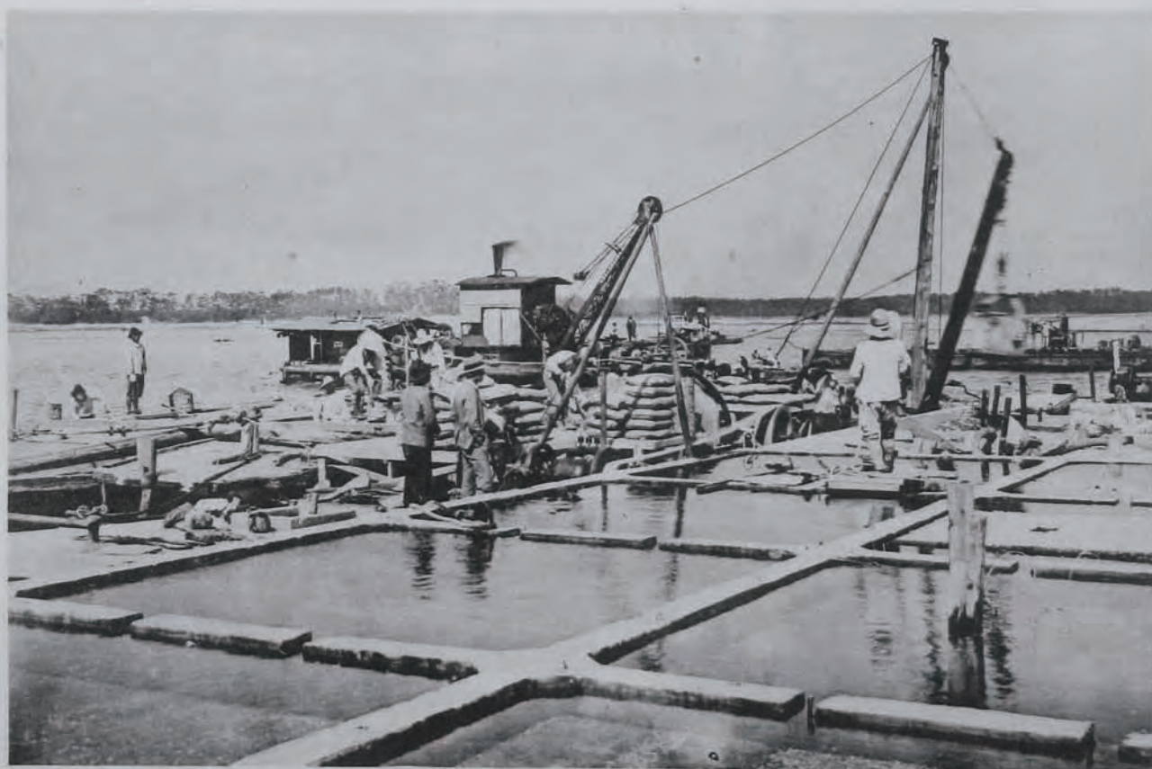
(28) 和歌山港修築工事南防波堤
