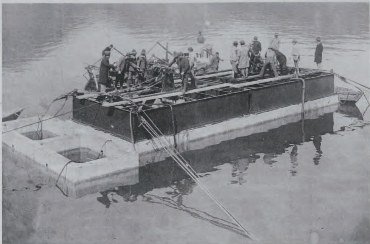
(27) 舞鶴港修築工事ケーソン据付作業
