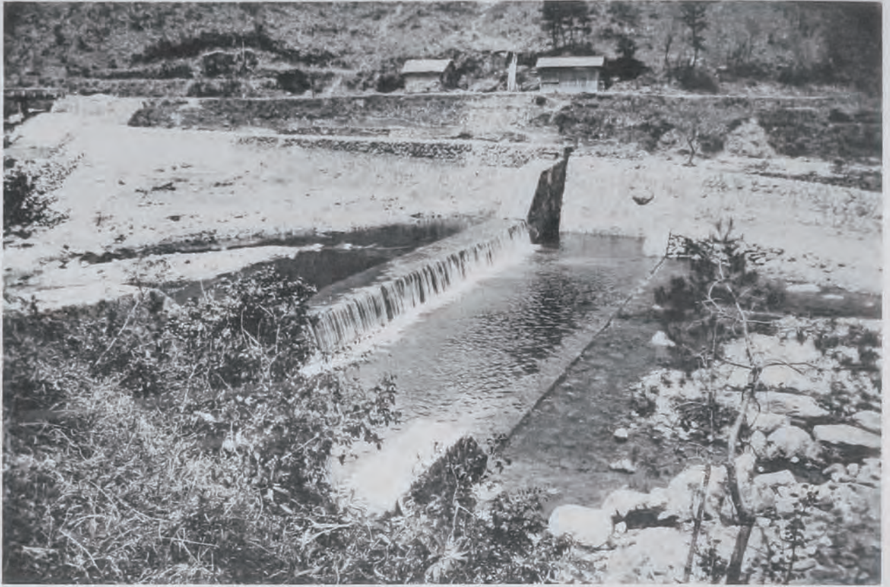
(19) 天神川改修工事竣功セル堰堤 (矢送川第一號堰堤右岸ヨリ望ム)
