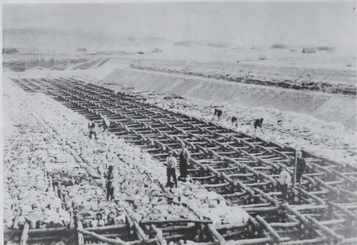
(3) 雄物川改修工事新川開鑿床固 (秋田縣河邊郡新屋町地内) 新川ノ床固ニ三層逆木床ヲ布設
