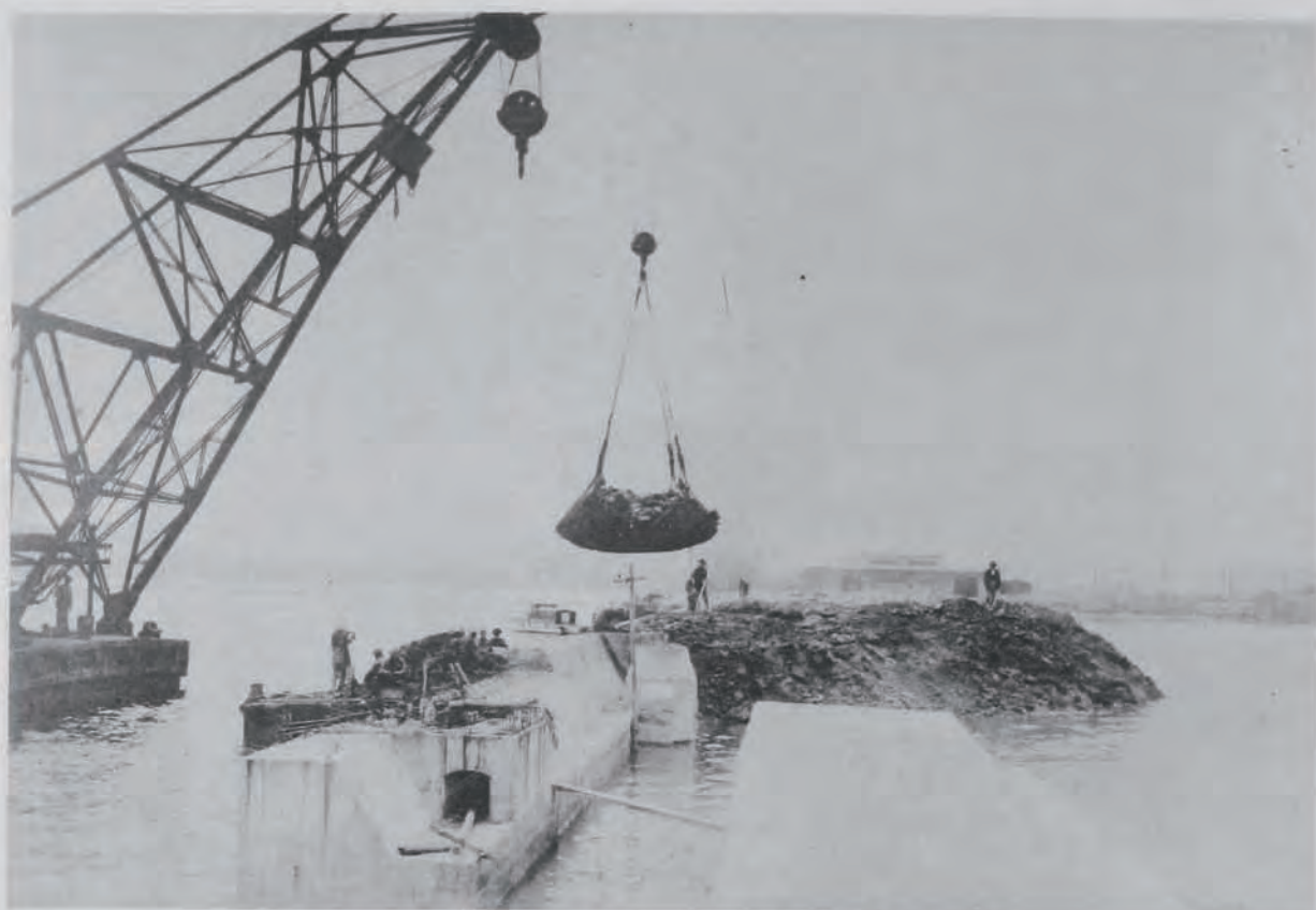
(19) 横濱港修築工事岸壁裏込状況 十米岸壁第二號工事
