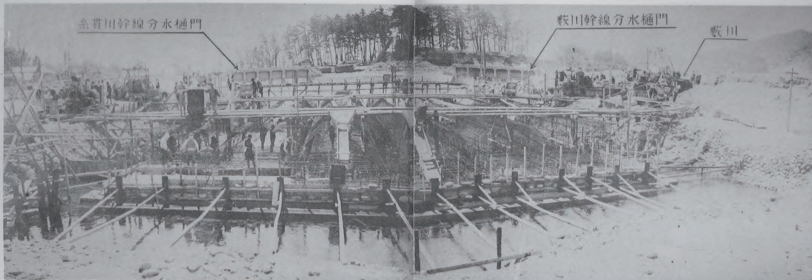
(1) 木曾川上流改修工事山口月水統一取水樋門床盤混凝土作業 (岐阜縣本巢郡山添村地并揖斐川支川藪川筋左岸) 樋門長二十三米、内法幅三米、高一米二(六連)
