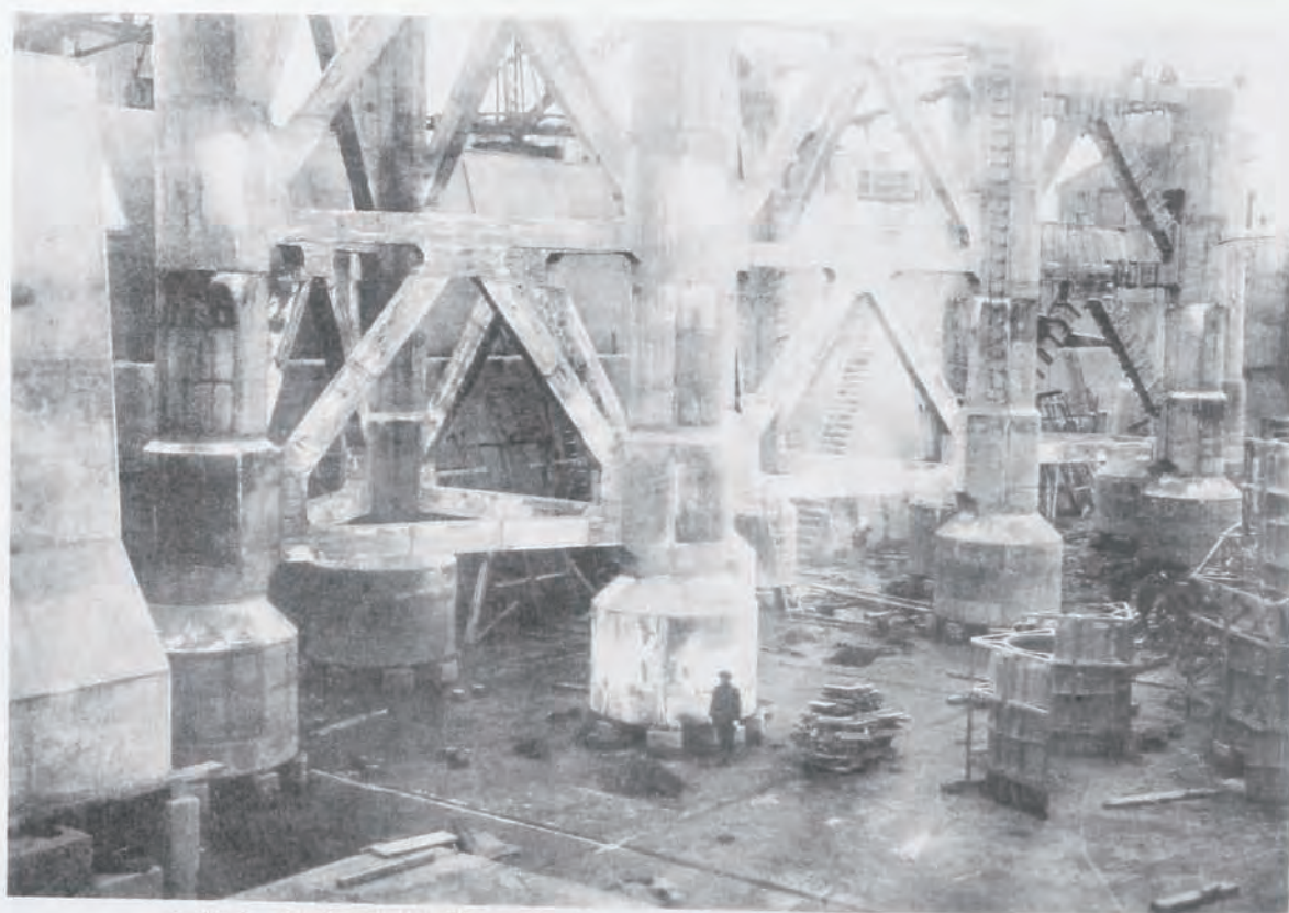
(46) 横濱港修築工事山下町棧橋補修用圓筒構製作 高十三米八、圓筒直徑下部三米、上部一米五、圓筒構ハ三個ノ圓筒ヨリ成ル
