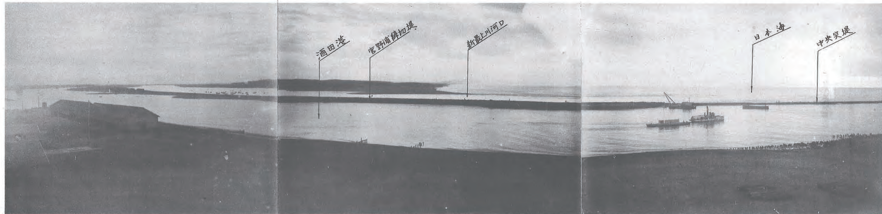
(2) 最上川改修工事宮野浦締切工事竣功後状況 (山形縣西田川郡袖浦村大字宮野浦地先)。
