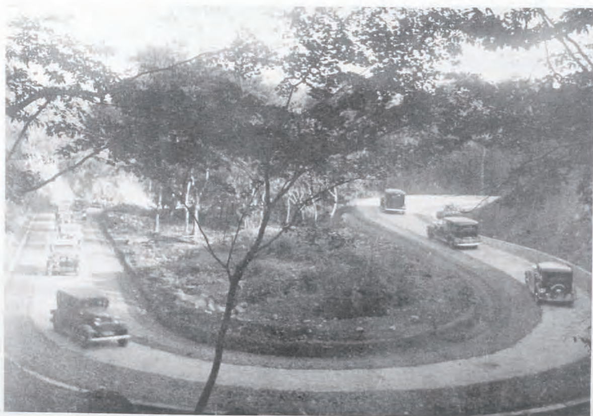
( 88 ) 國道十號線(碓氷)國道改良工事改良後ノ狀況 (群馬縣碓氷郡坂本町地内) 中央幅員三米混凝土鋪裝
