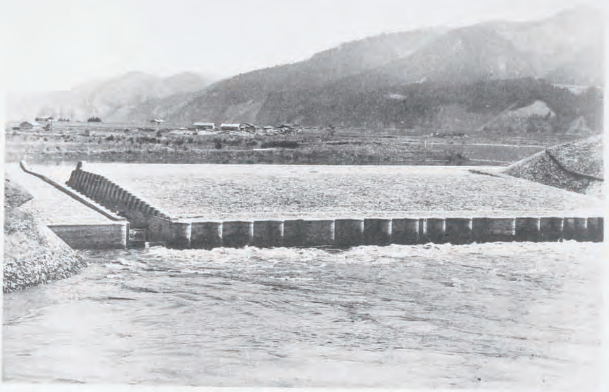
( 9 ) 北上川改修工事 嶋波洗堰 魚道 (宮城縣遠田郡豊里村地先) 溢流部幅三米ヲ切り下ゲ魚道トス
