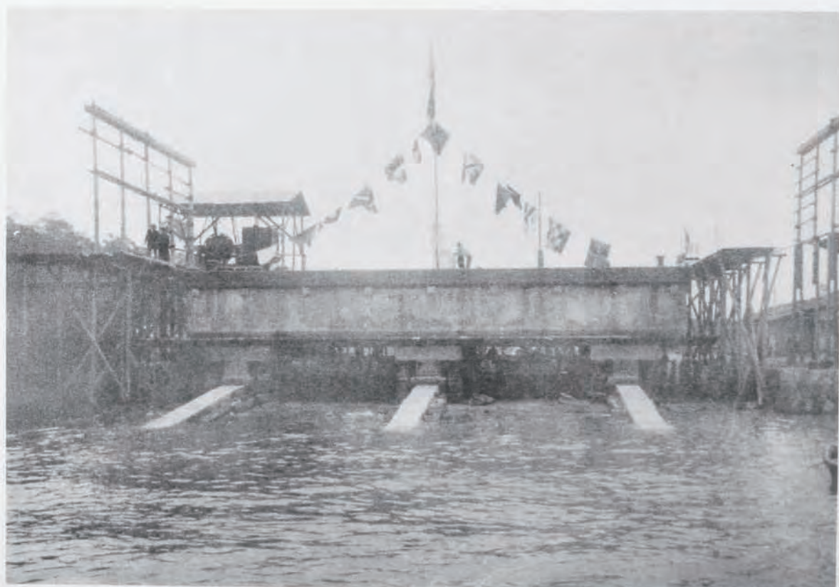
(56) 尾道港修築工事棧橋用浮函 浮函長二十米、幅八米、高二米六
