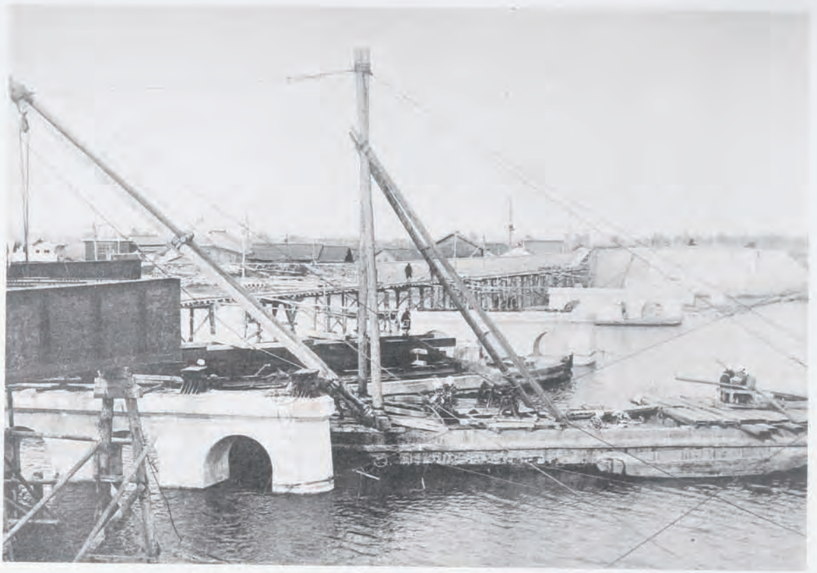
(65) 國道一號線(名古屋)改良工事三日月橋 (愛知縣愛知郡下ノ一色町及海部郡富田村地内) 新川ニ架ス、全長百五十五米、徑間三十三米三連、 二十四米二連、有効幅員十一米、車道八米、歩道各一米五
