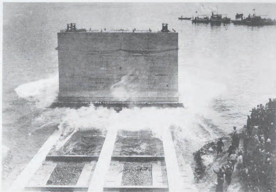
(55) 宮古港修築工事防波堤ケーソン進水 ケーソン長十四米、上幅四米五、下幅八米六、高七米八
