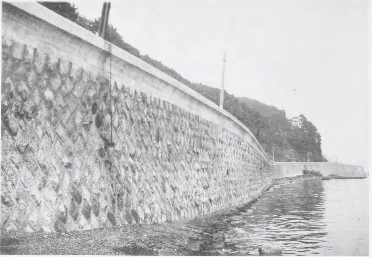
( 77 ) 國道三號線(大分)改良工事石積擁壁 (大分縣大分郡八幡村地内)
