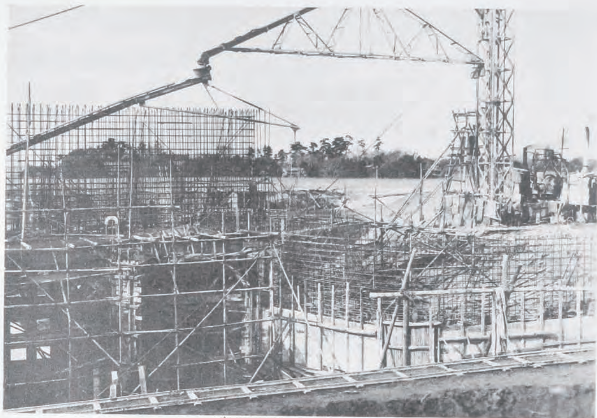
(13) 木曾川上流改修工事境川樋門 (岐阜縣羽島郡小龍村地先) 幅五米、高七米、四連
