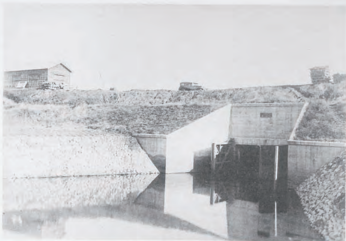
(15) 木曾川上流改修工事論田樋門 (岐阜縣稻葉郡日置江村地先) 幅三米、高三米、二連
