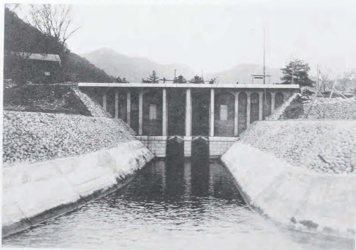
(18) 木曾川上流改修工事忠節用水取水樋門 (岐阜縣岐阜市地先) 幅一米六、高二米六、二連
