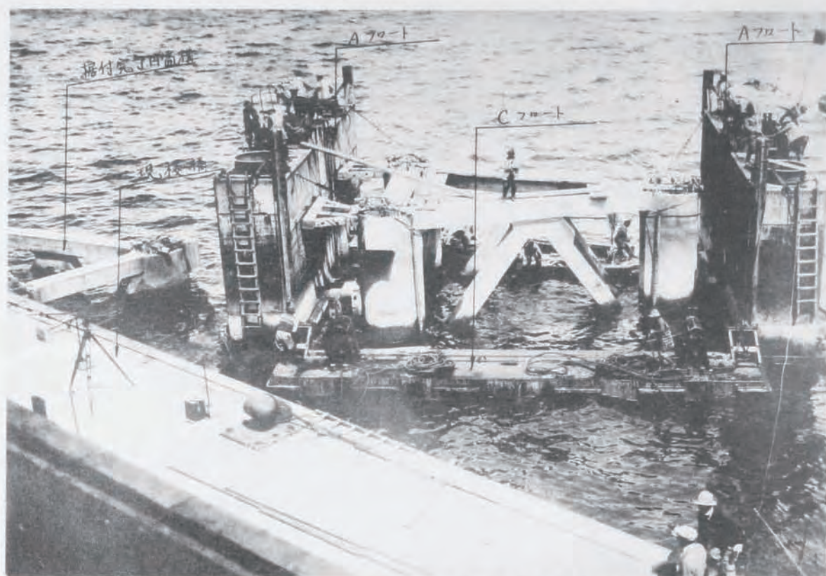
(47) 横濱港修築工事山下町棧橋補修用圓筒構据付 圓筒構重量二百噸、フロート浮力百二十噸
