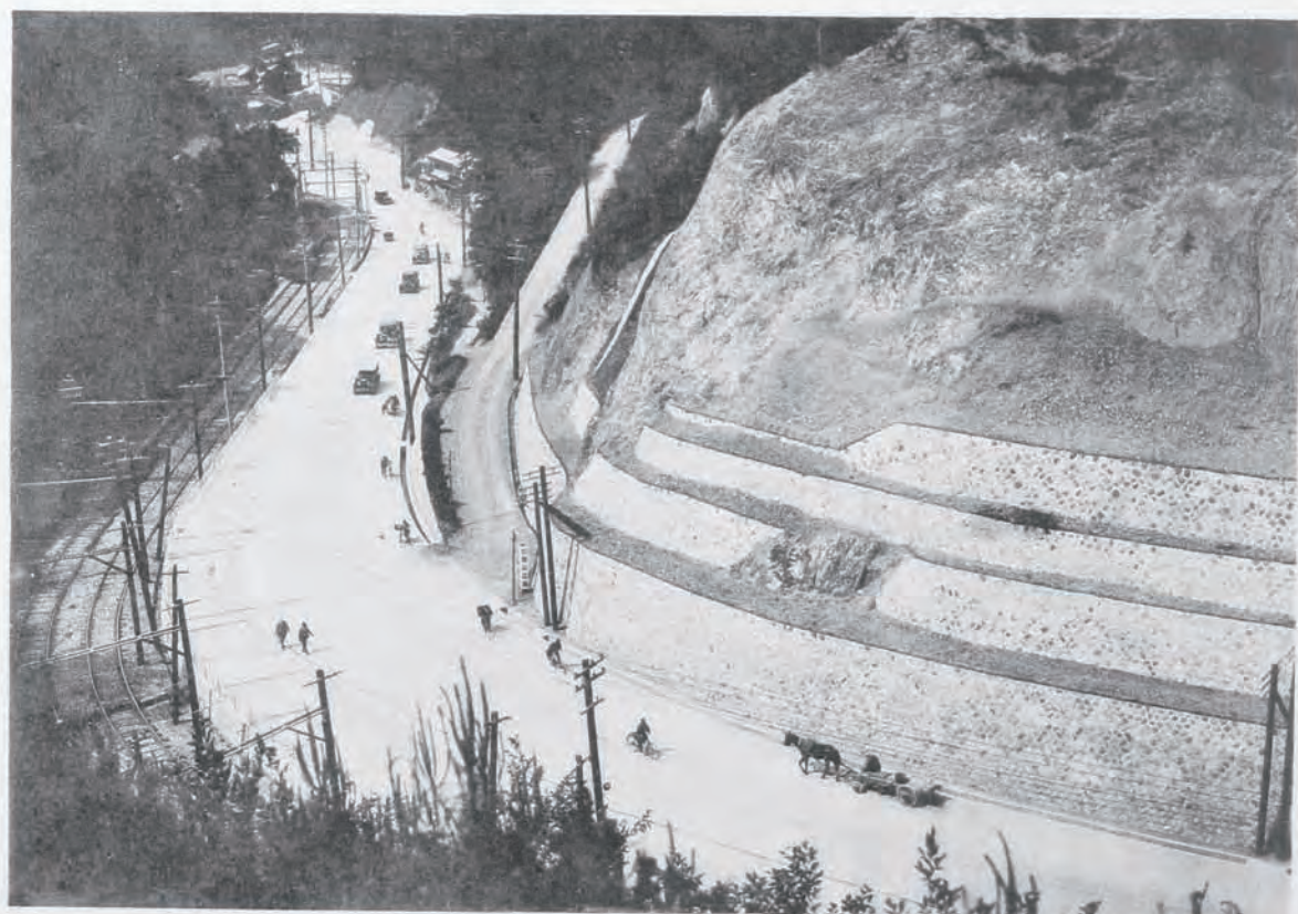
(72) 國道二號線(京都)改良工事新道路 其一 (京都市東山區山科日ノ岡地内)
