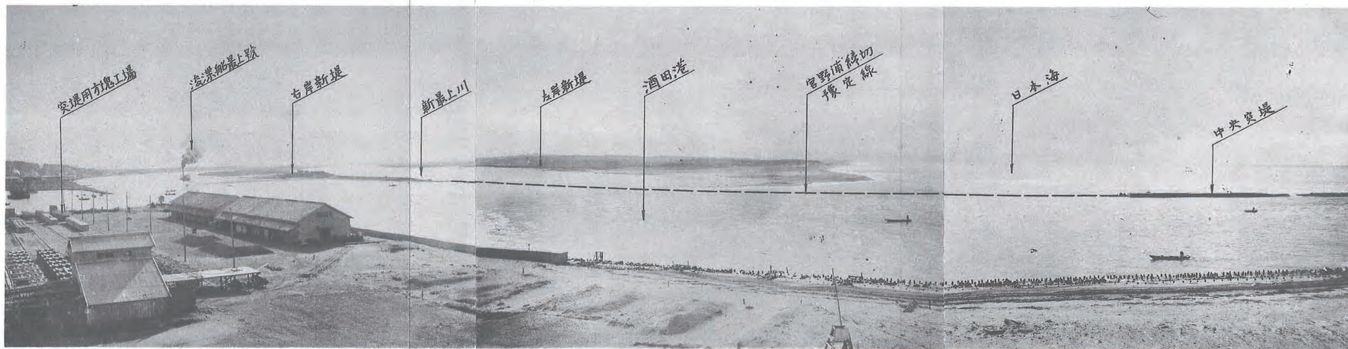
(1) 最上川改修工事宮野浦締切工事着手前状況 (山形縣西田川郡袖浦村大字宮野浦地先)。
