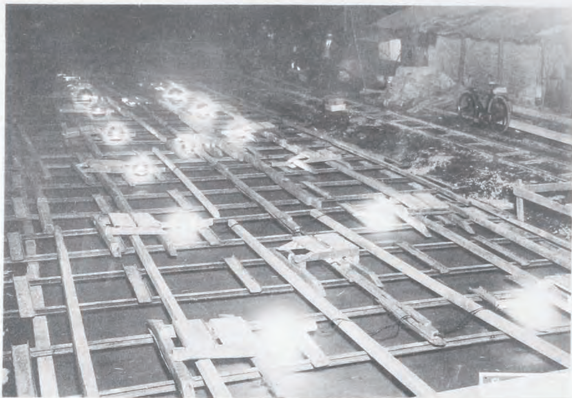
(81) 国道六號線(金町)改良工事混凝土保温装置
