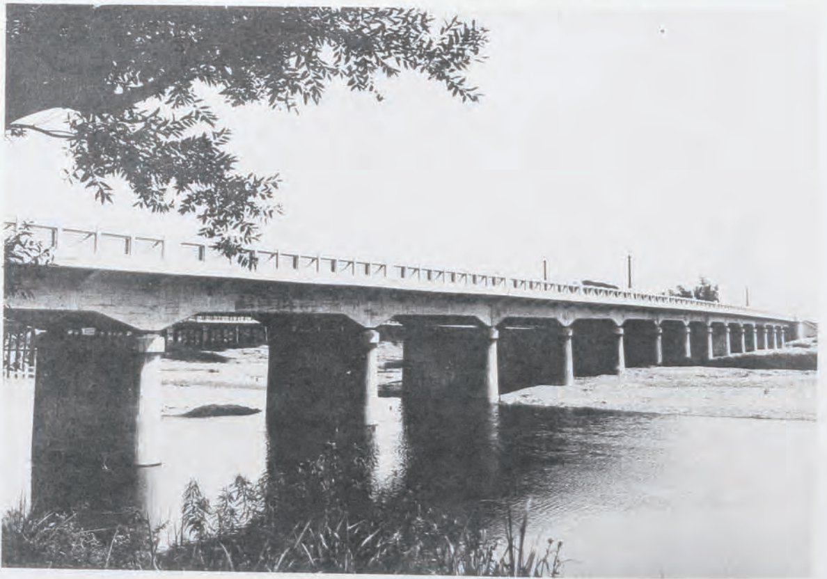
(66) 國道一號線(桑名)改良工事町屋橋 其一 (三重縣桑名郡城南村及三重郡朝日村地内) 町屋川ニ架ス、全長二百十四米六、有効幅員七米五
