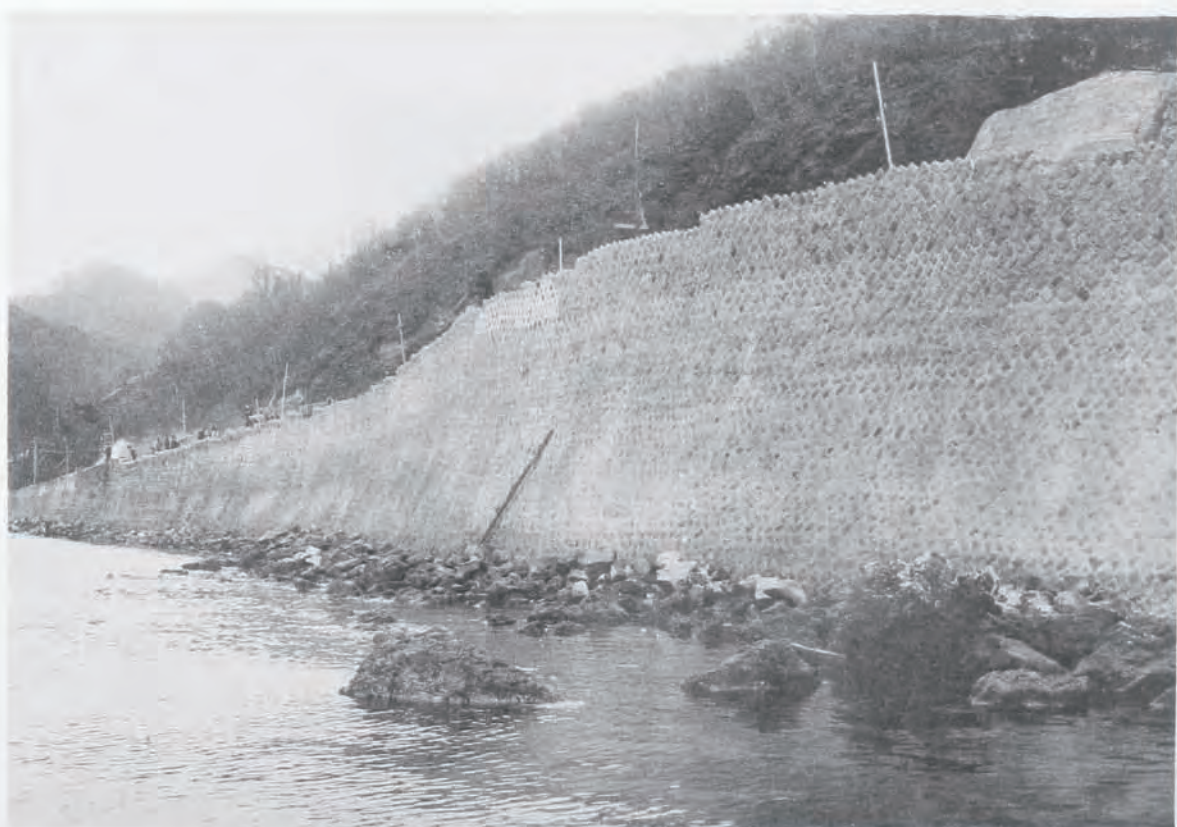
( 80 ) 國道四號線(青森)改良工事金山跨線橋附近擁壁 (青森縣東津輕郡野内村浅虫地内)
