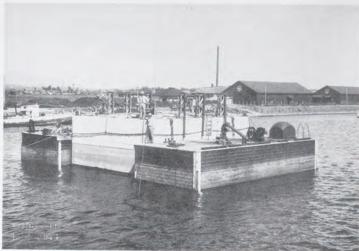
(53) 土崎港修築工事突堤用面運搬 其二 面ヲフロートニテ浮カシ吃水ヲ二米トス
