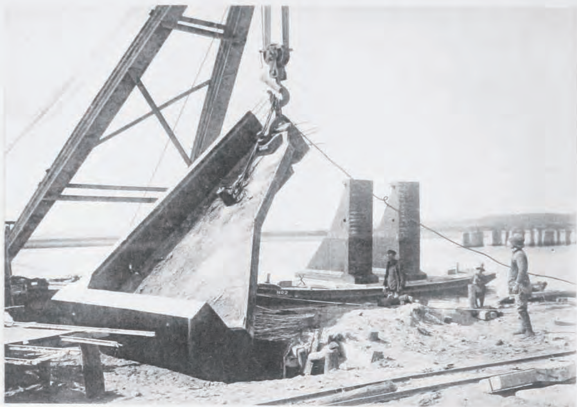
(3) 最上川改修工事酒田護岸用塊運搬
