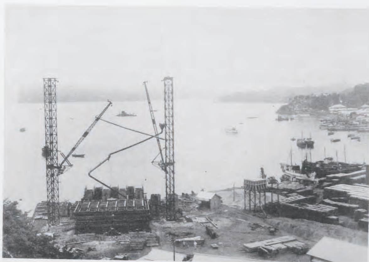
(54) 宮古港修築工事ケーソン製作場
