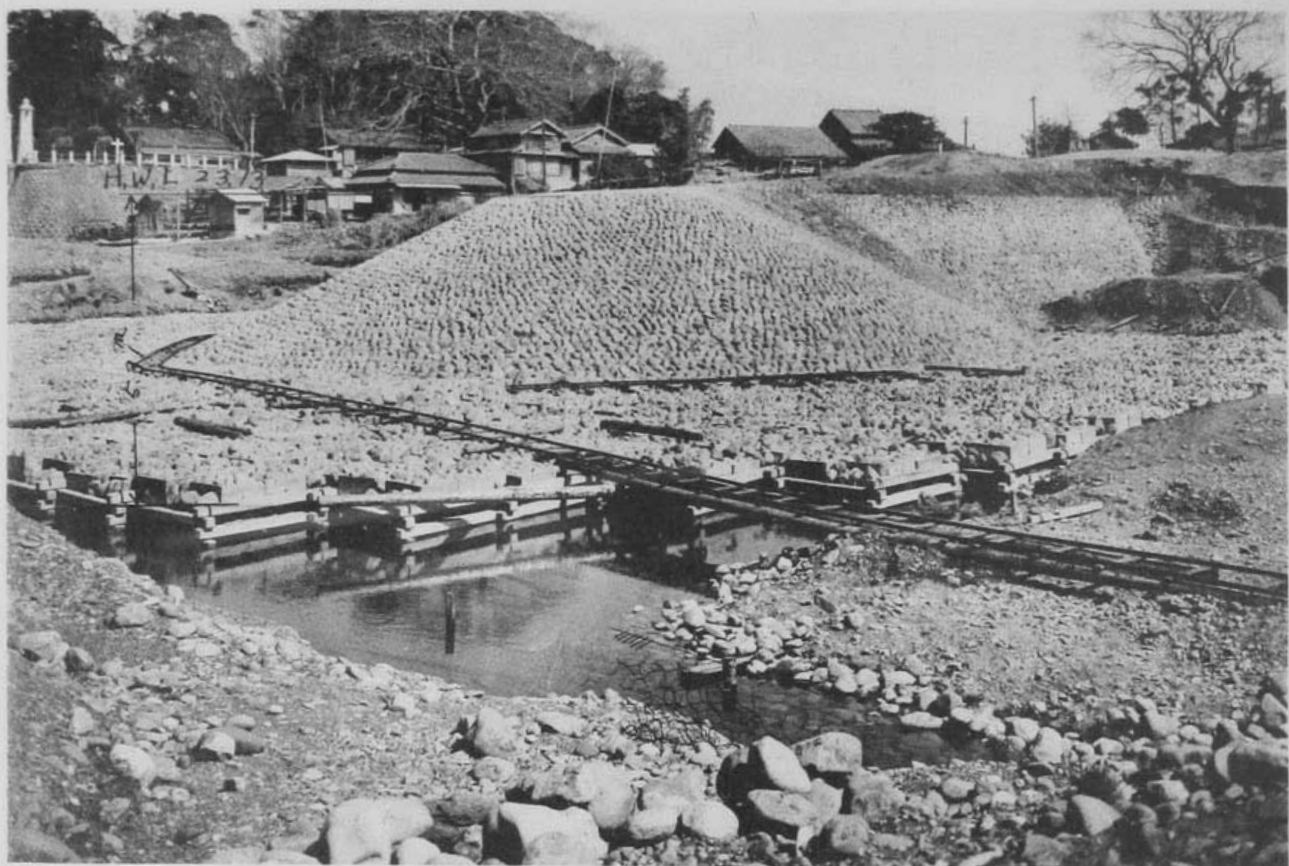
(7) 富士川改修工事下流水神一番水制 (静岡縣富士郡岩松村大字松岡地先、延長三十三米)
