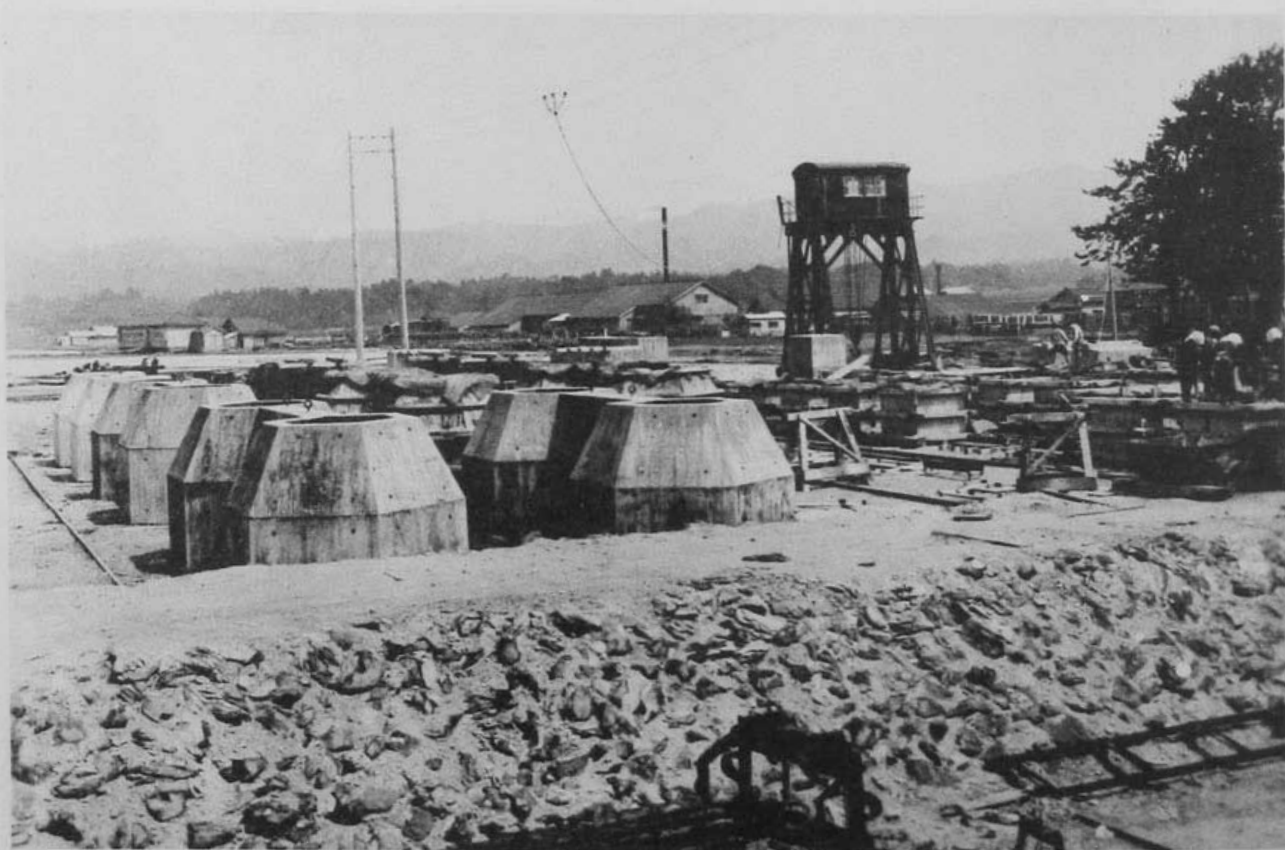
(28) 七尾港修築工事混凝土作業場 (石川県鹿島郡七尾町大字矢田新、東湊村大字萬行 地先、棧橋用基礎沓、落岸、防波堤用方塊製作)
