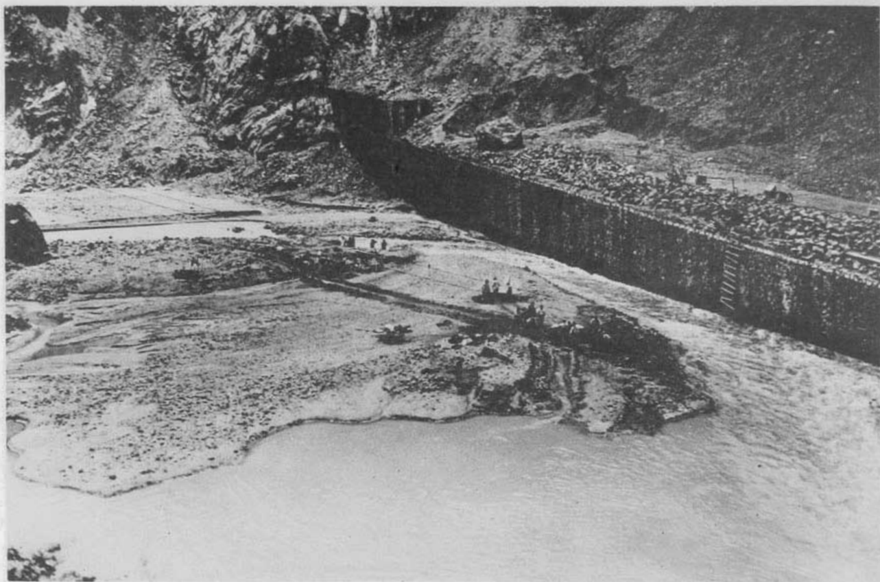
(15) 常願寺川砂防工事堰堤背後砂礫貯積 (富山縣上新川郡大山村大字有峰、中新川郡立山村大字蘆峯寺地先)
