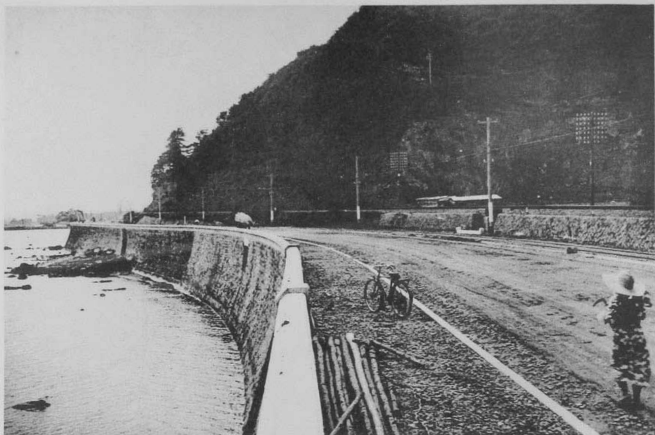
( 37 ) 國道三號線(大分)改良工事竣功道路 (大分縣大分郡八幡村大字神崎地内起點一號乃至七年度終點附近)
