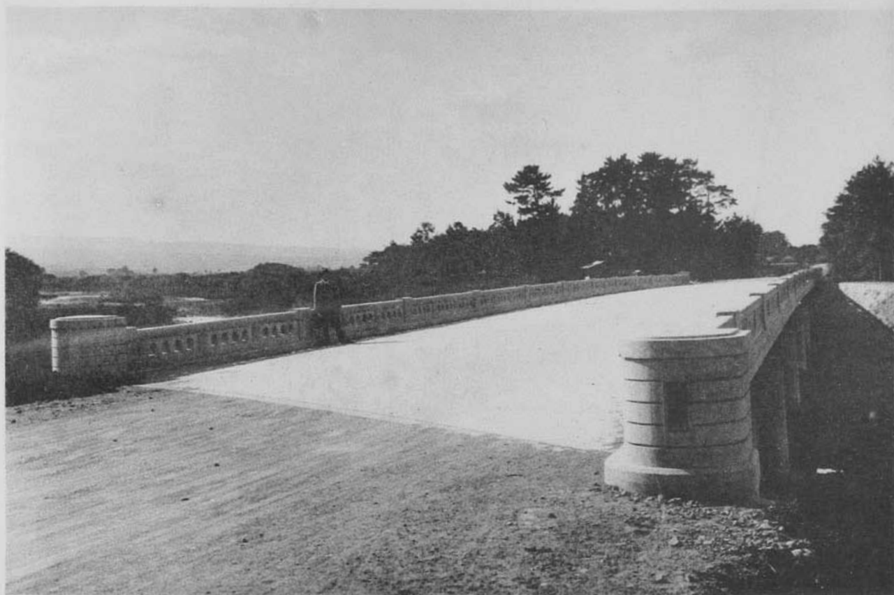
( 39 ) 國道三號線(八屋)改良工事竣功セル佐井川橋 (主桁鐵筋組立完了狀況)
