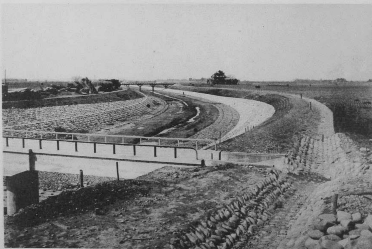
( 2 ) 最上川改修工事内川新放水路 (鶴岡市大字道形地先、掛樋附近ヨリ下流ヲ望ム)
