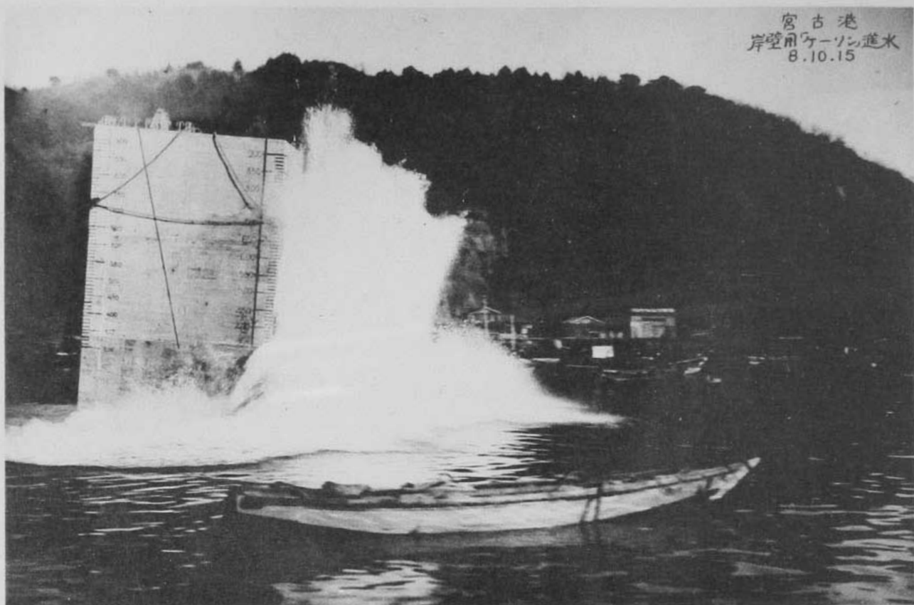
(27) 宮古港岸壁用「ケーソン」進水状況 (ケーソン長十四米〇六、上幅五米五、下幅七米五、高九米四、重量約五百六十吨)
