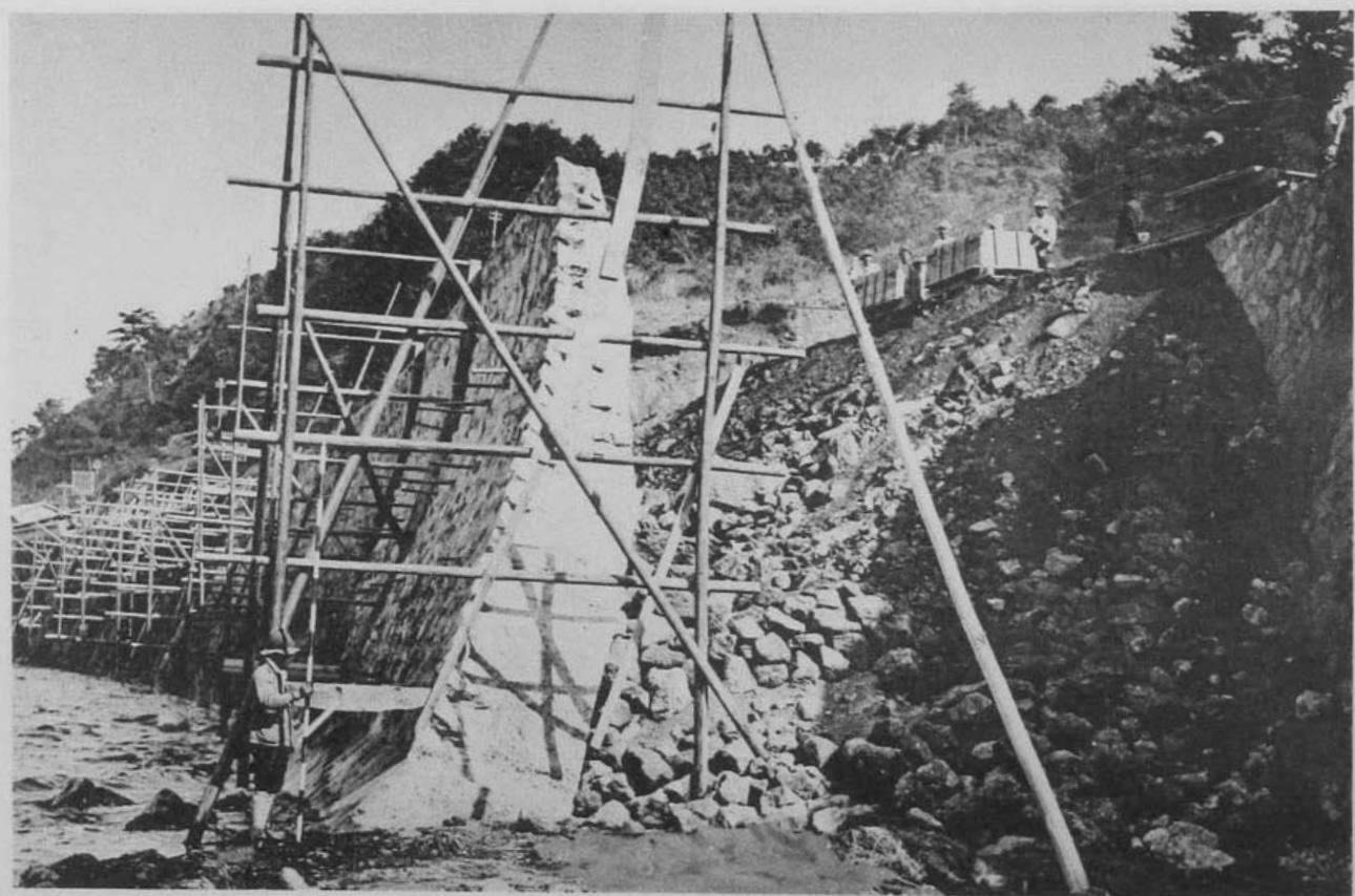
( 36 ) 國道三號線(大分)改良工事作業狀況 (大分縣大分郡八幡村大字神崎地内起點一號乃至七年度終點附近)
