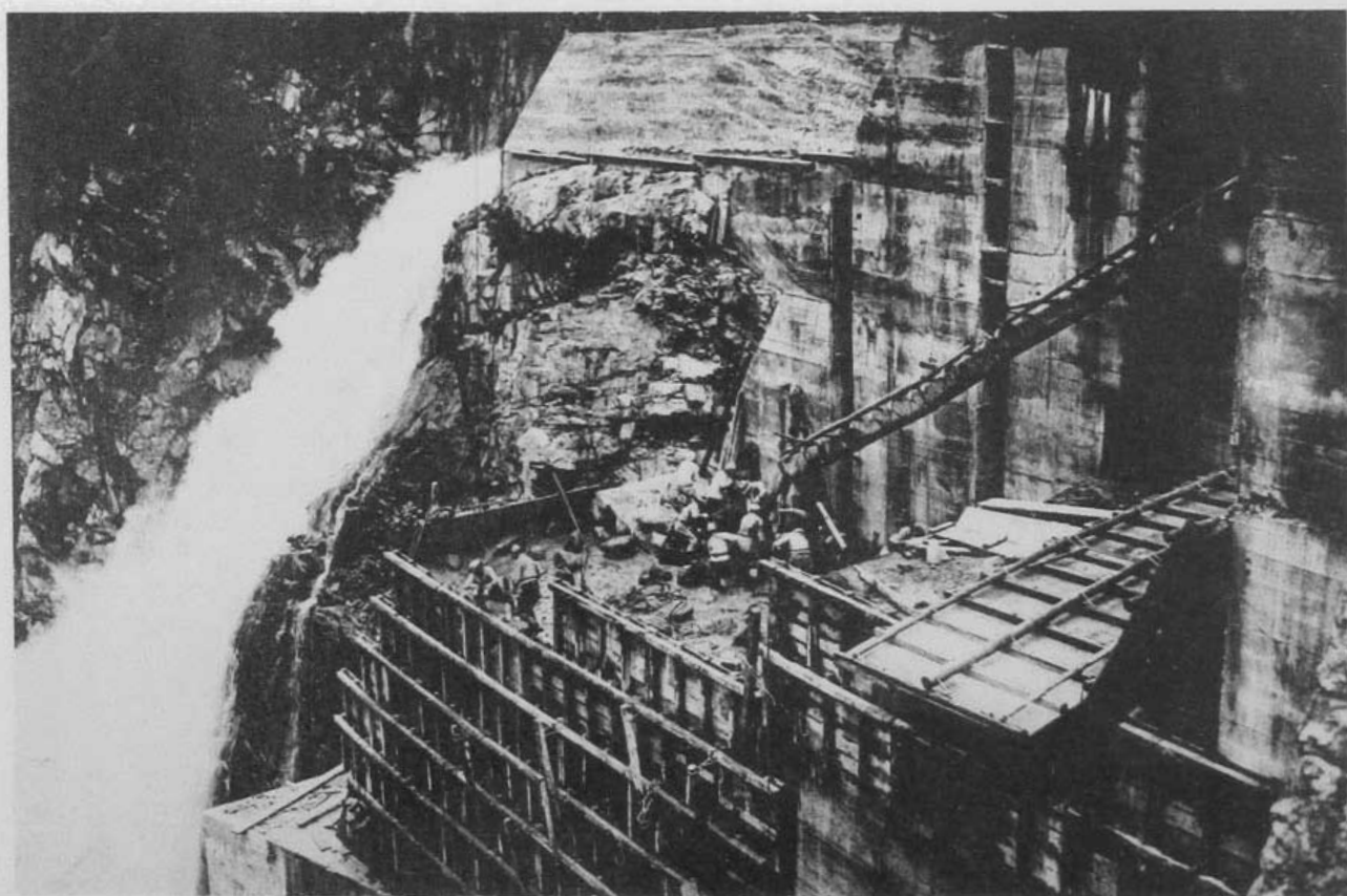
(16) 常願寺川砂防工事白岩堰堤混凝土作業 (富山縣中新川郡立山村大字蘆峯寺、上新川郡大山村大字有峰地先)
