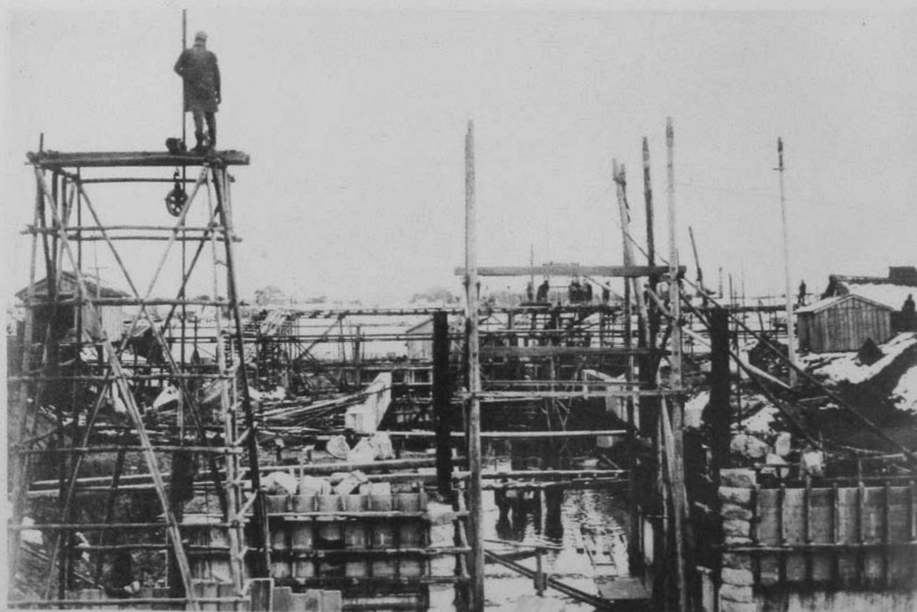
(4) 神通川改修工事萩之浦閘門 (富山縣婦負郡草島村地先、矢板打込及閘門室混凝土打作業)
