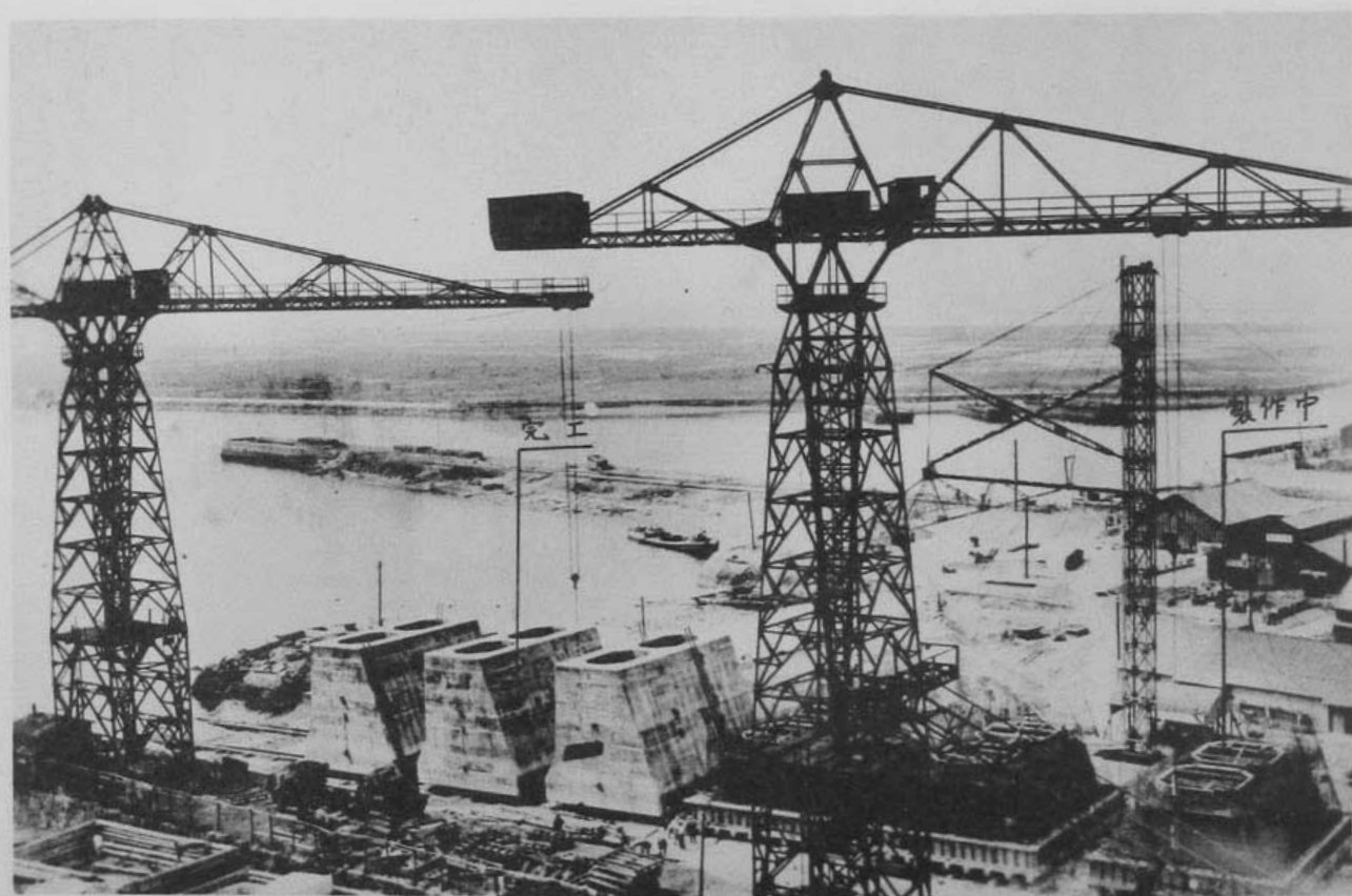
(20) 横濱港修築工事函塊製作 (鶴見工場ニ於ケル製作状況)
