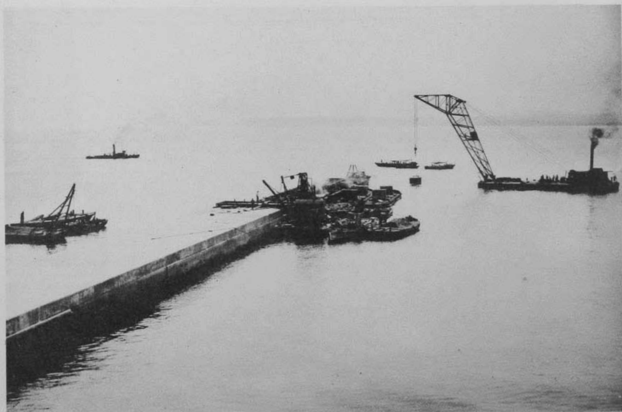
( 26 ) 小名濱港修築工事防波堤築造作業 (堤頂部混凝土及方塊据付作業)
