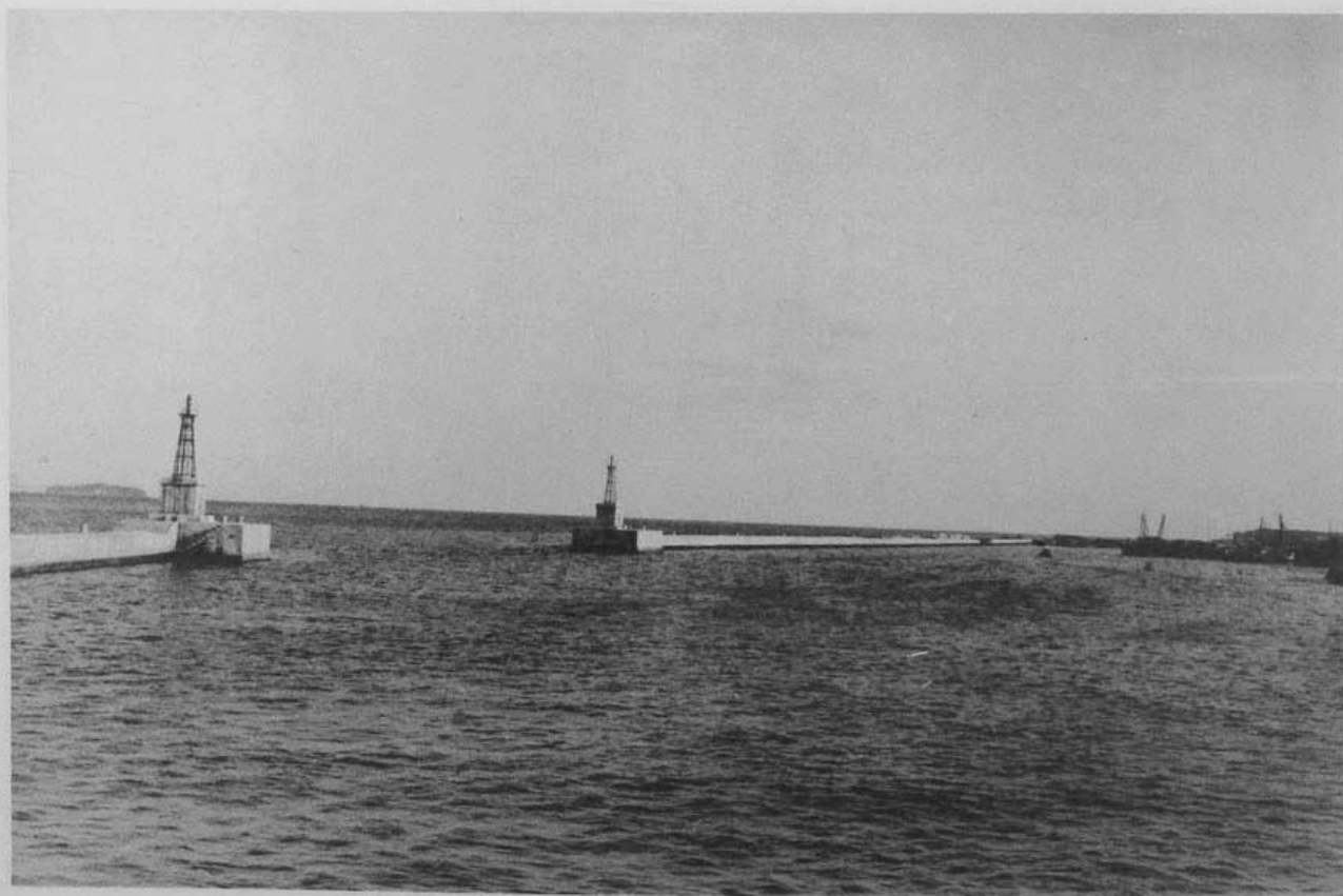
(22) 鹿兒島港修築工事南北兩防波堤 (港内ヨリ港外ヲ望ム)
