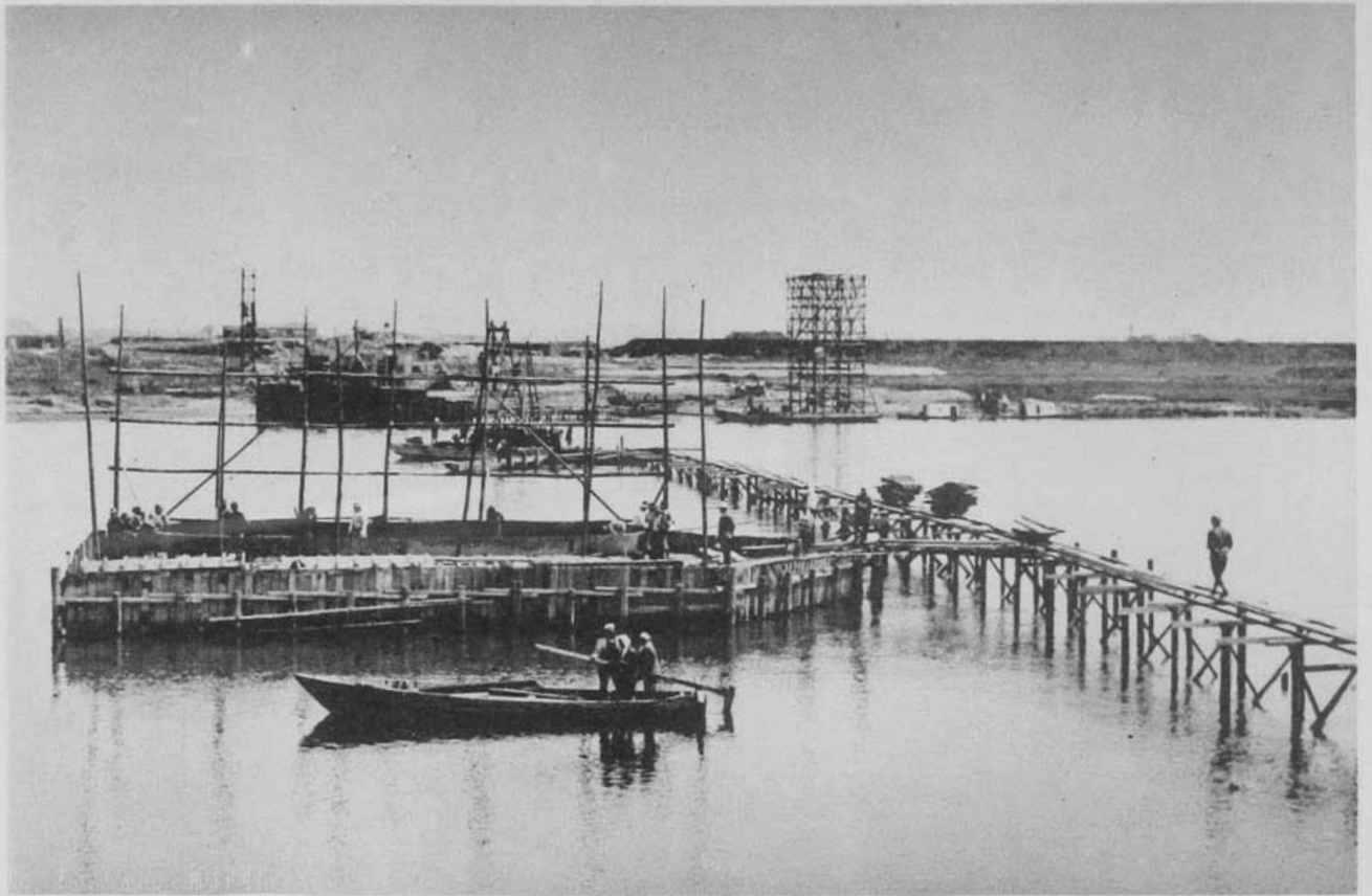
( 45 ) 國道十號線(秋田)改良工事雄物川橋脚井筒 (秋田市牛島町及河邊郡新屋町百三段新屋地内)
