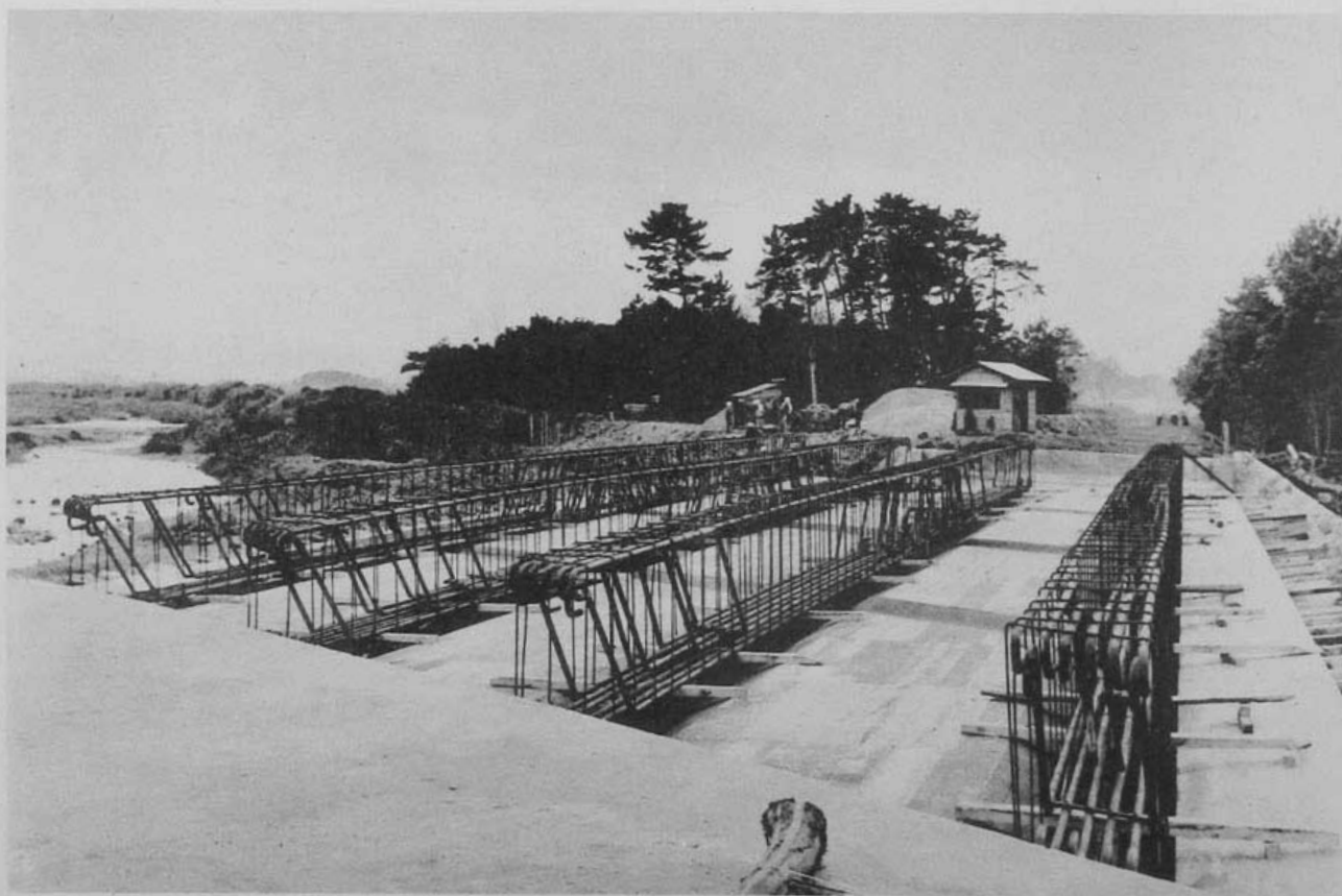
( 38 ) 國道三號線(八屋)改良工事組立中ノ佐井川橋 (主桁鐵筋組立完了狀況)
