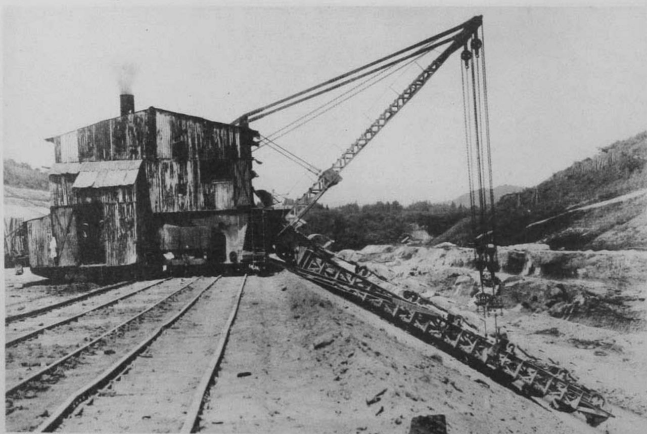
( 6 ) 阿賀川改修工事袋原掘鑿 (福島縣河沼郡川西村地先、長梯掘鑿機下掘ノ狀況、 ロングラッター長十五米、バケット二十九個、一個ノ 容積〇・二六立方米、能力十時間ニ付一千二百立方米)
