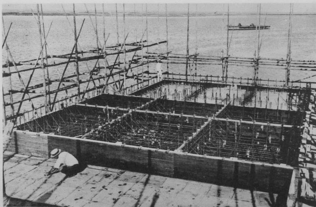
(24) 土崎港修築工事突堤用函塊底部鐵筋配置 (函塊方五米五、幅七米五、長十米)
