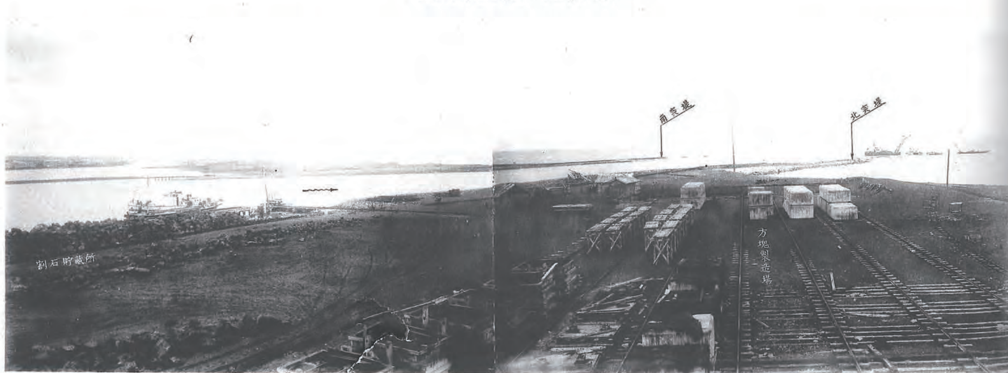
(4) 岩木川改修工事十三湖水戸口突堤 (青森縣西津輕郡十三村地先) 南突堤延長百七十米、北突堤延長百七十米
