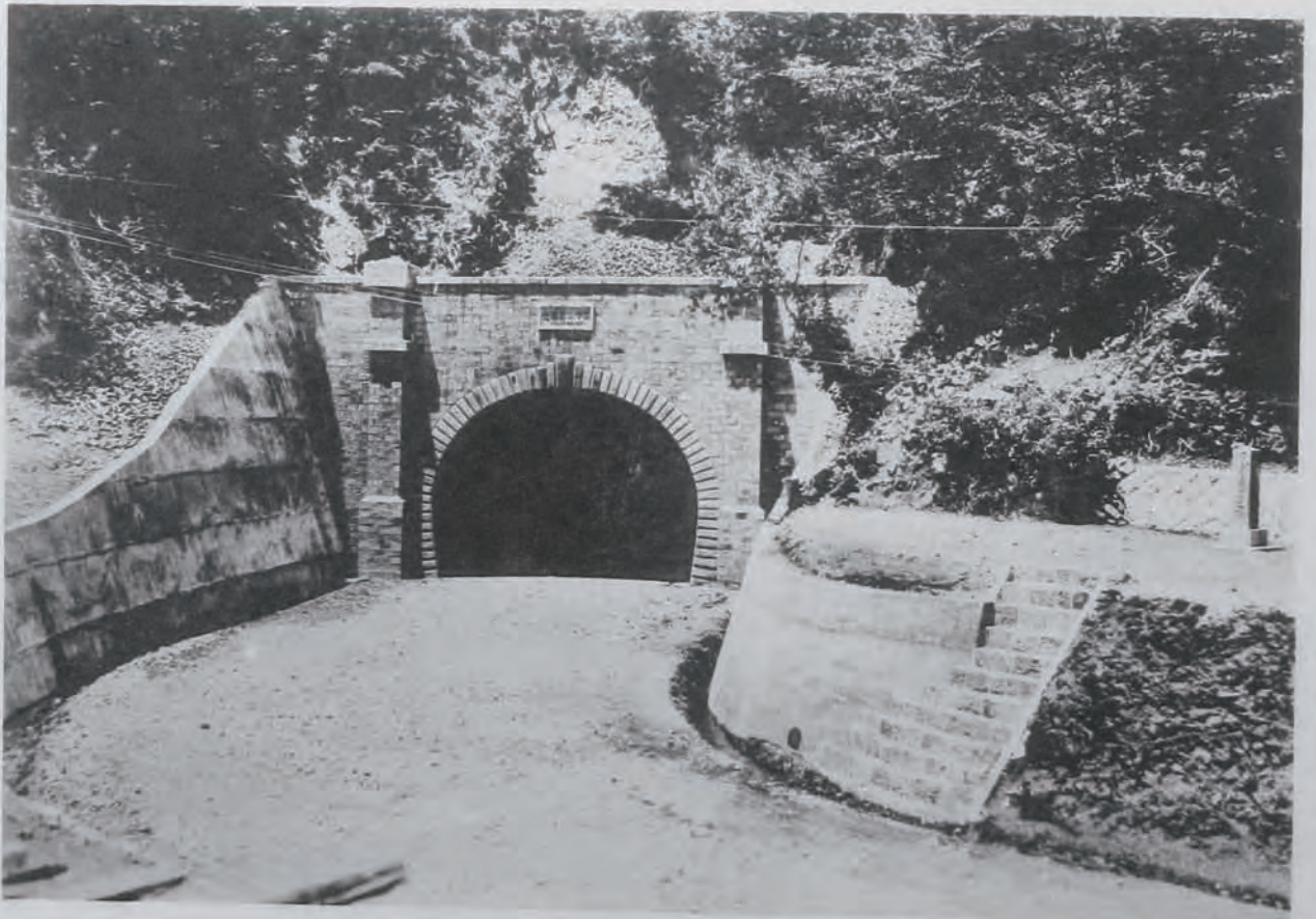
( 47 ) 國道五號線(福島)改良工事竣功セルニツ小屋隧道南口 (福島縣信夫郡中野村地内) 隧道延長三百八十四米、厚五十糎乃至四十糎、混凝土卷立、有効 幅員六米、有効高四米五、拱型高五米〇四、路面混凝土鋪裝
