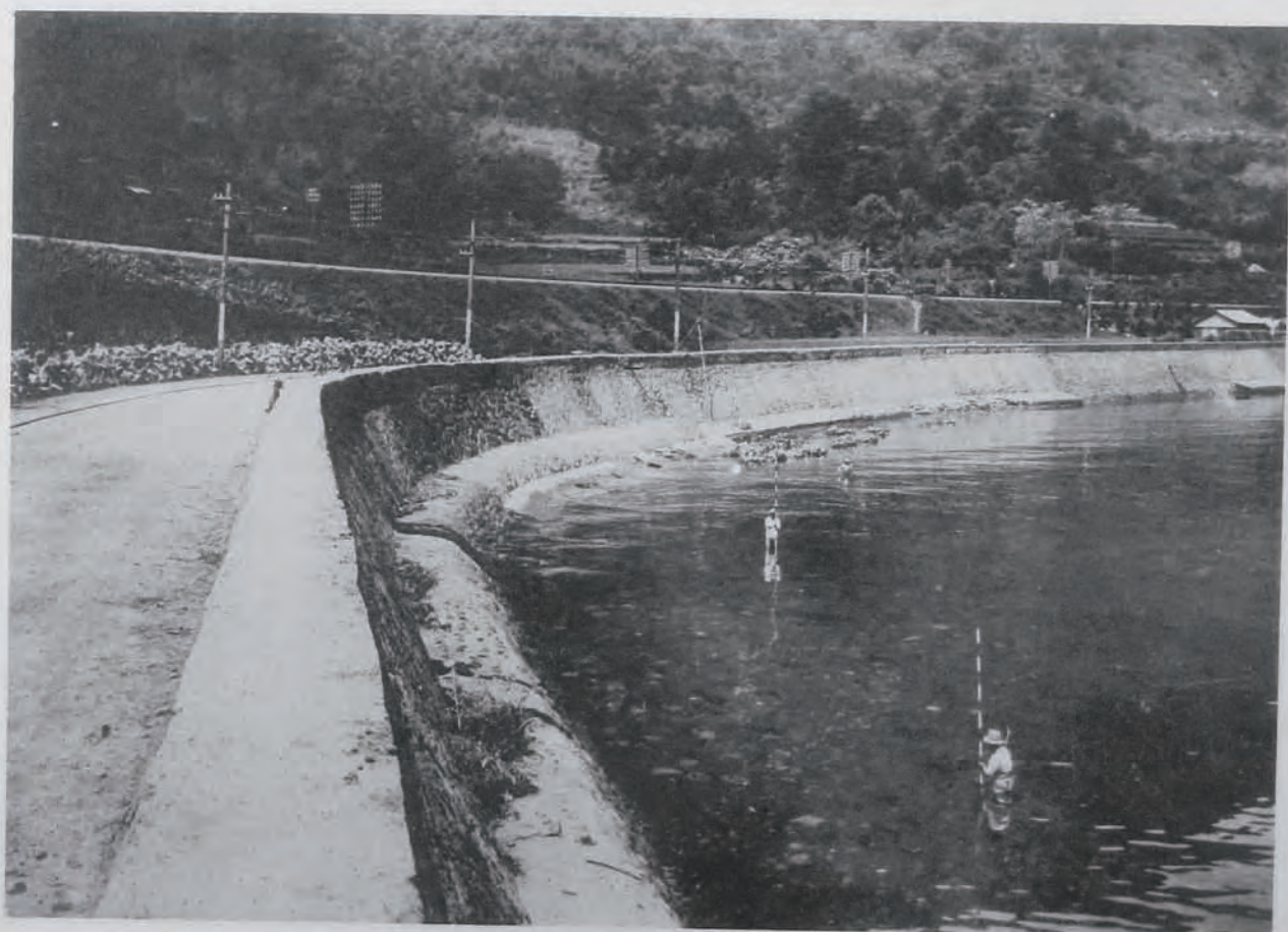
( 43 ) 國道三號線(大分)改良工事海岸實測 (測點四十號乃至五十號附近)
