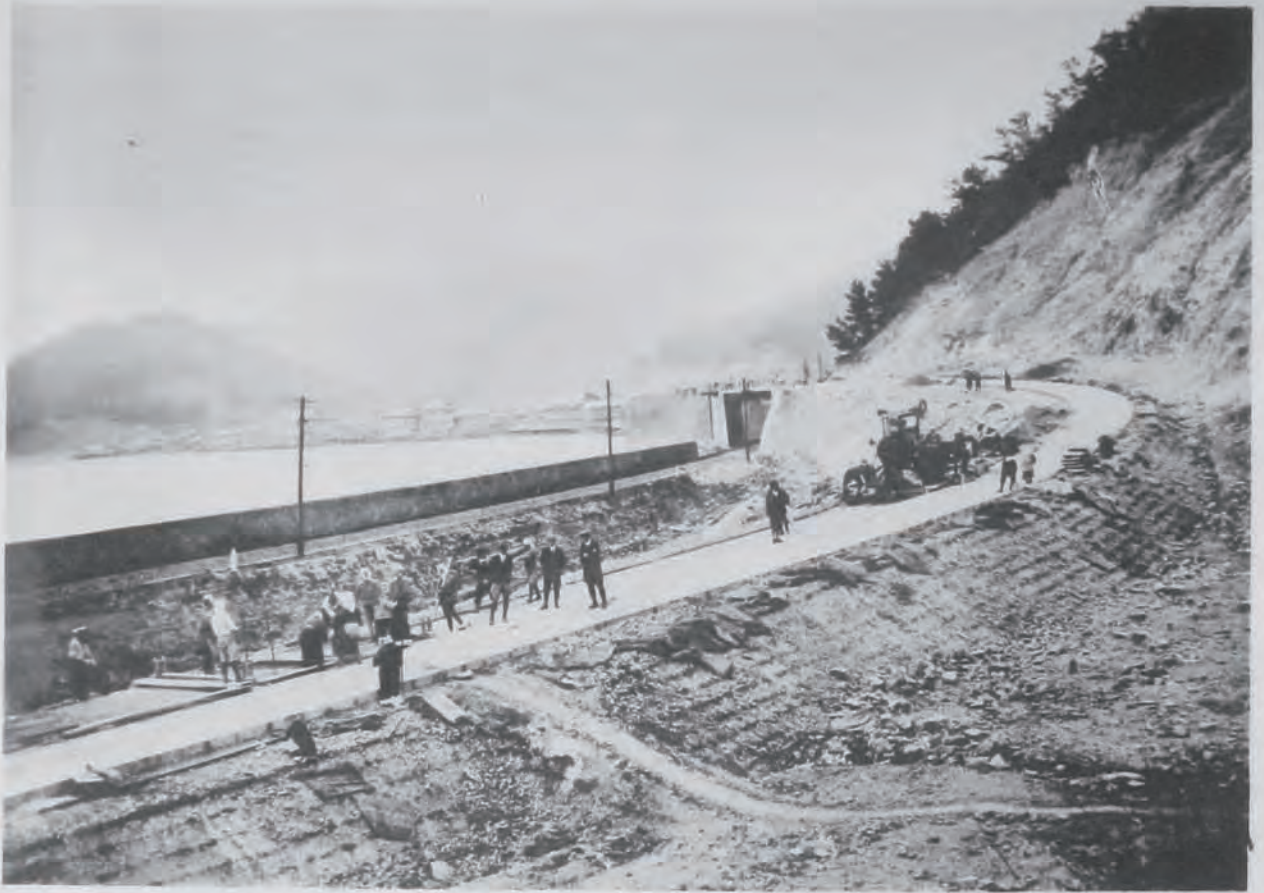
( 46 ) 國道四號線(青森)改良工事混凝土鋪裝作業 (青森縣東津輕郡野内村大字浅虫地内) 鋪 裝 幅 員 六 米
