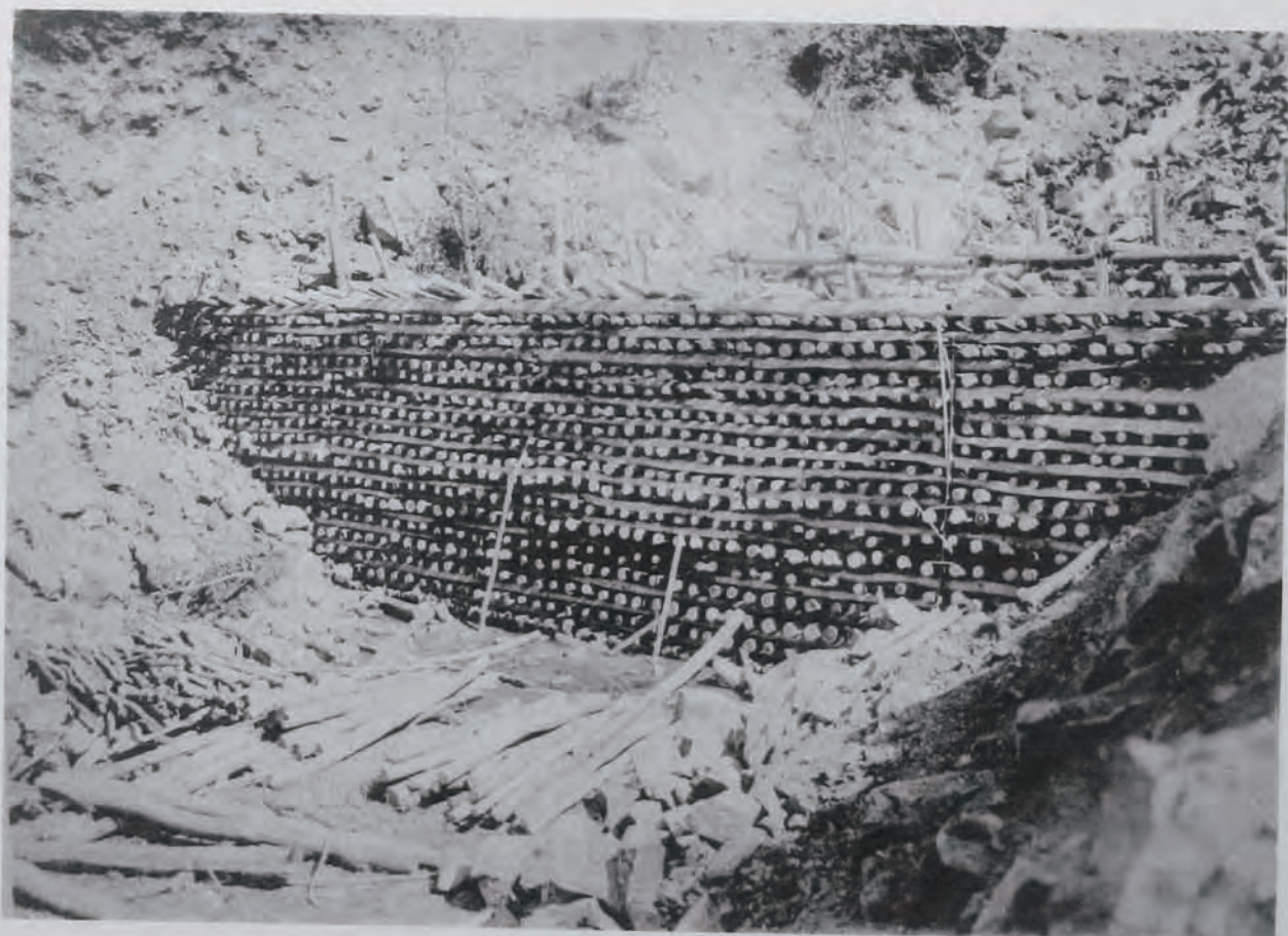
(21) 揖斐川砂防工事黒谷假木造堰堤 (岐阜縣吉城郡上寶村大字一重ヶ根地内) 假木造堰堤施工中
