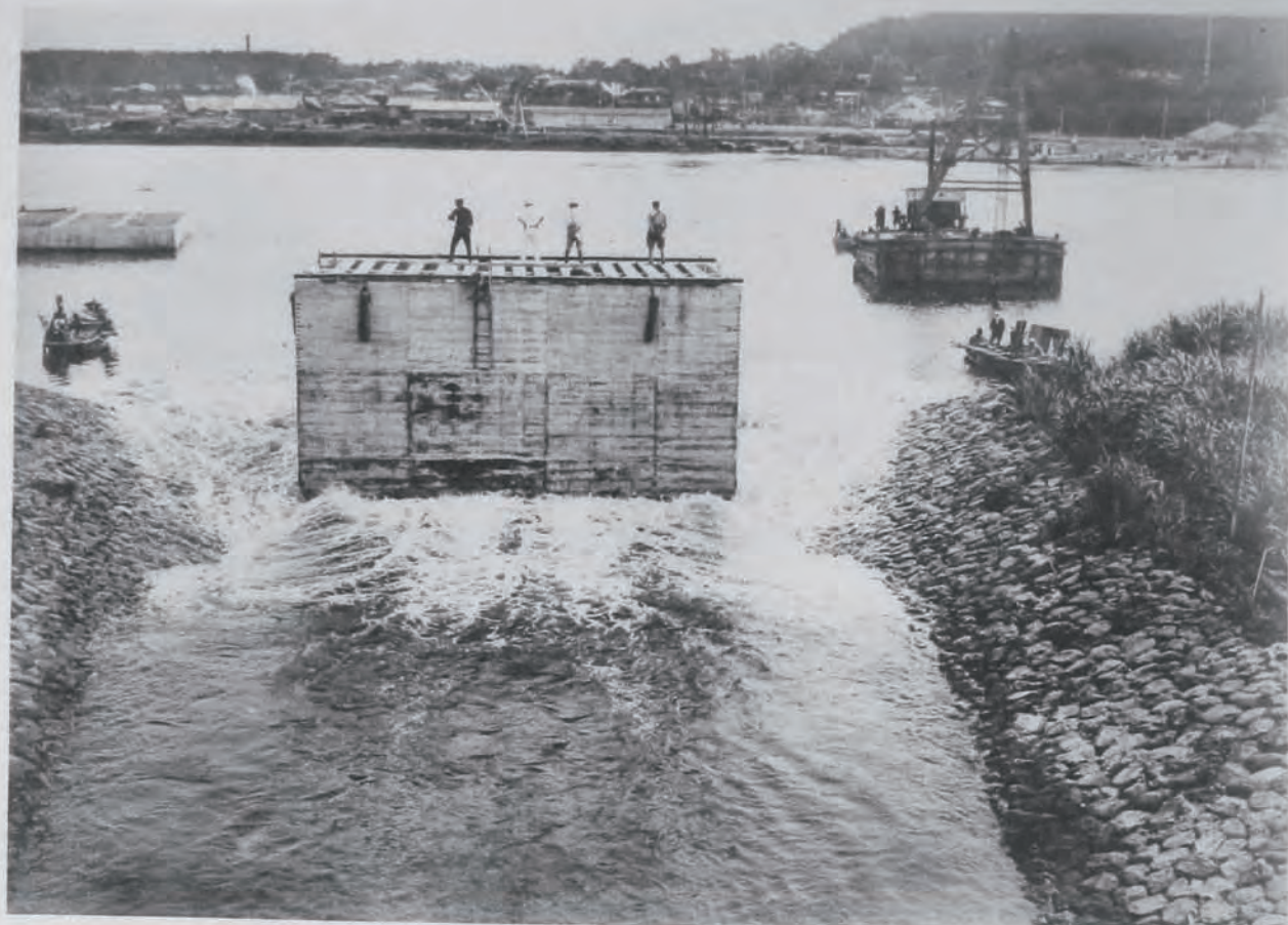
( 36 ) 酒田港修築工事防波堤工事函塊進水 酒田市字下瀬修船架
