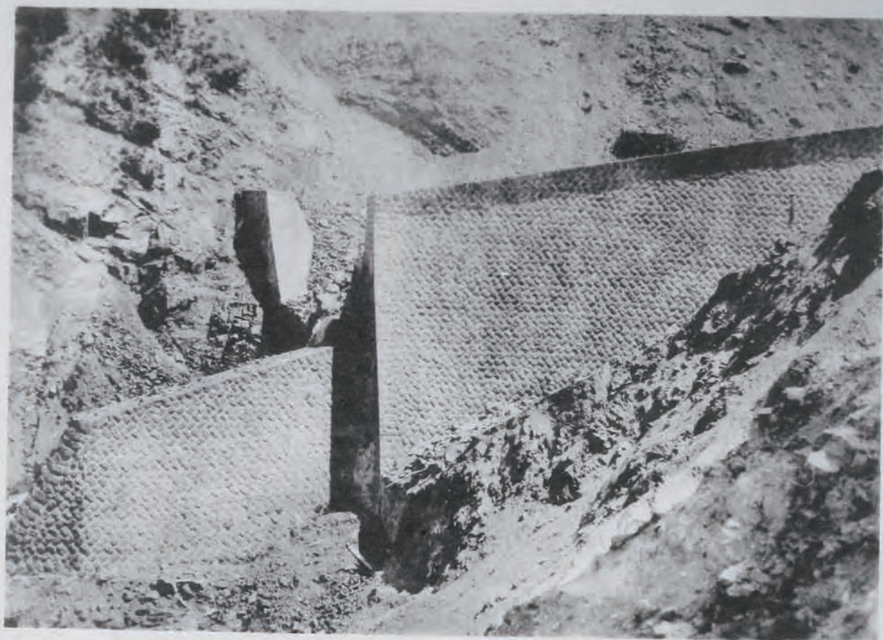
(20) 揖斐川砂防工事黒谷第一號護岸 (岐阜縣吉城郡上寶村大字中尾地内) 護岸嵩置及増築變更工事
