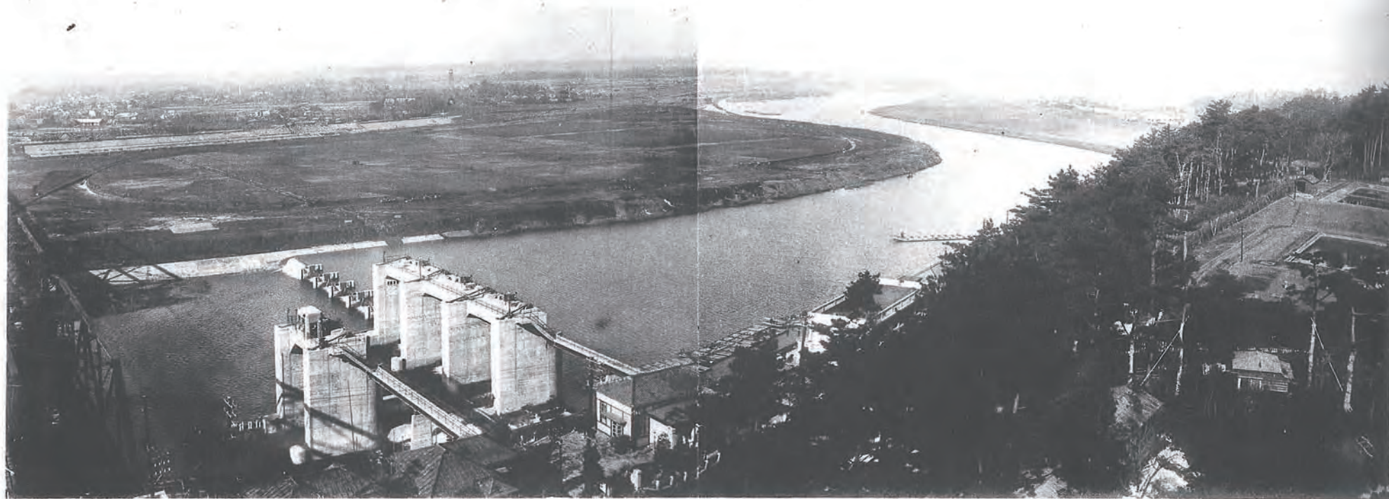
(3) 多摩川改修工事丸子橋附近展望 多摩川圖展望塔上ヨリ上流ヲ望ム
