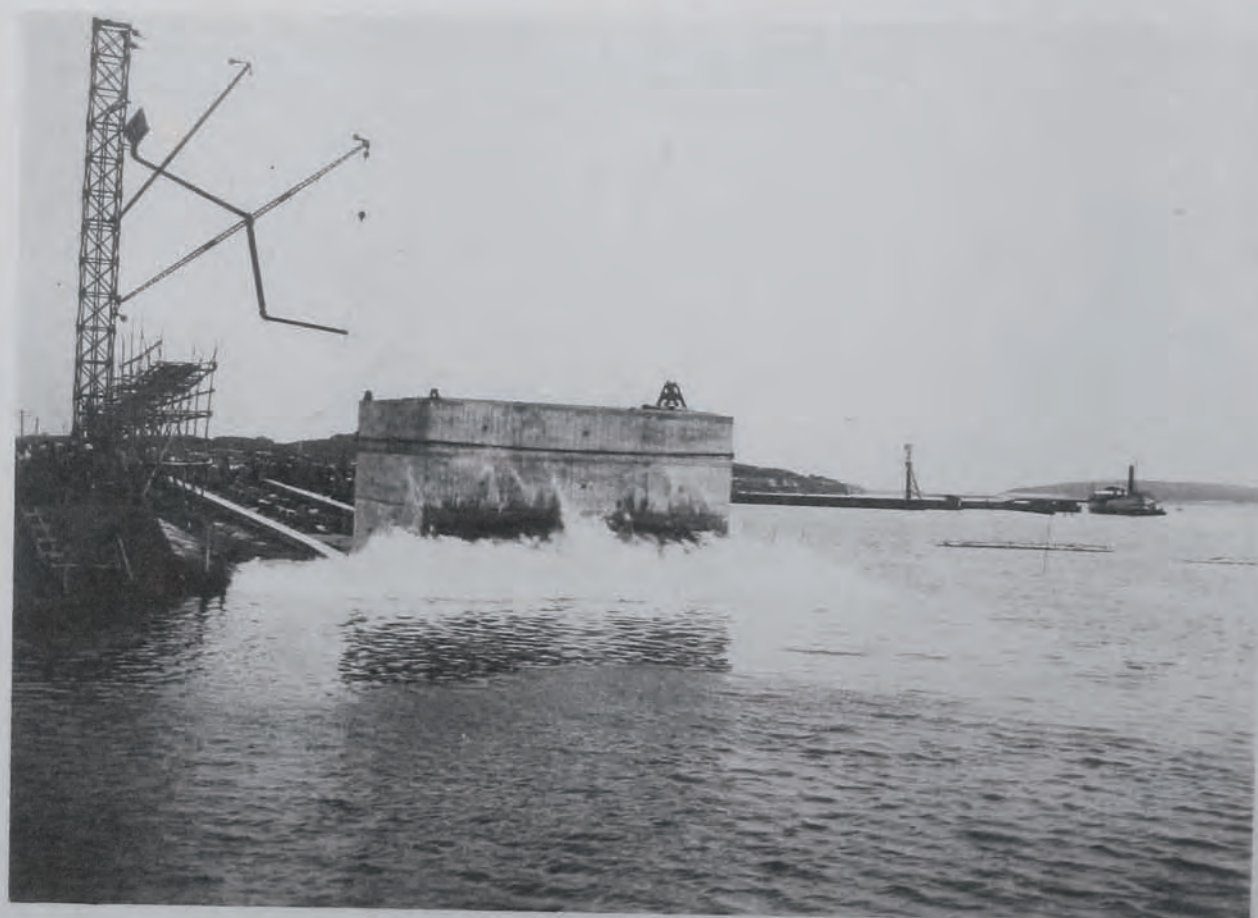
(27) 土崎港修築工事突堤用函塊 函塊進水ノ狀況、函塊長十米、幅七米五、高五米五
