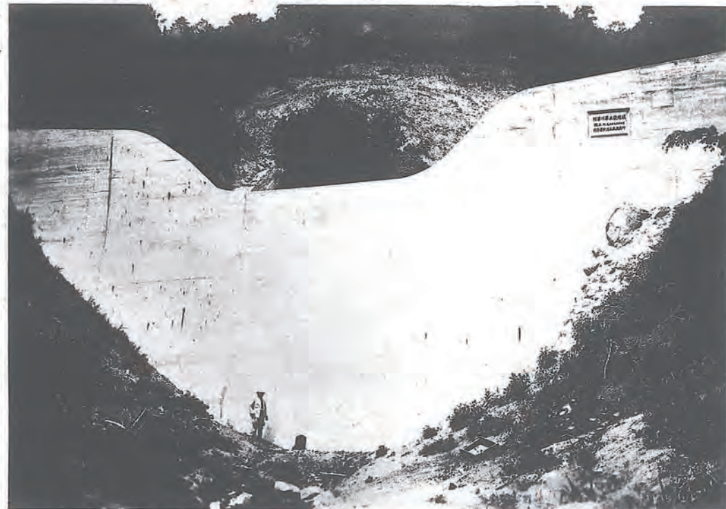
(12) 信濃川水系砂防工事檜澤川第三堰堤 (長野縣北安曇郡廣津村地内) 左岸下流ヨリ望ム
