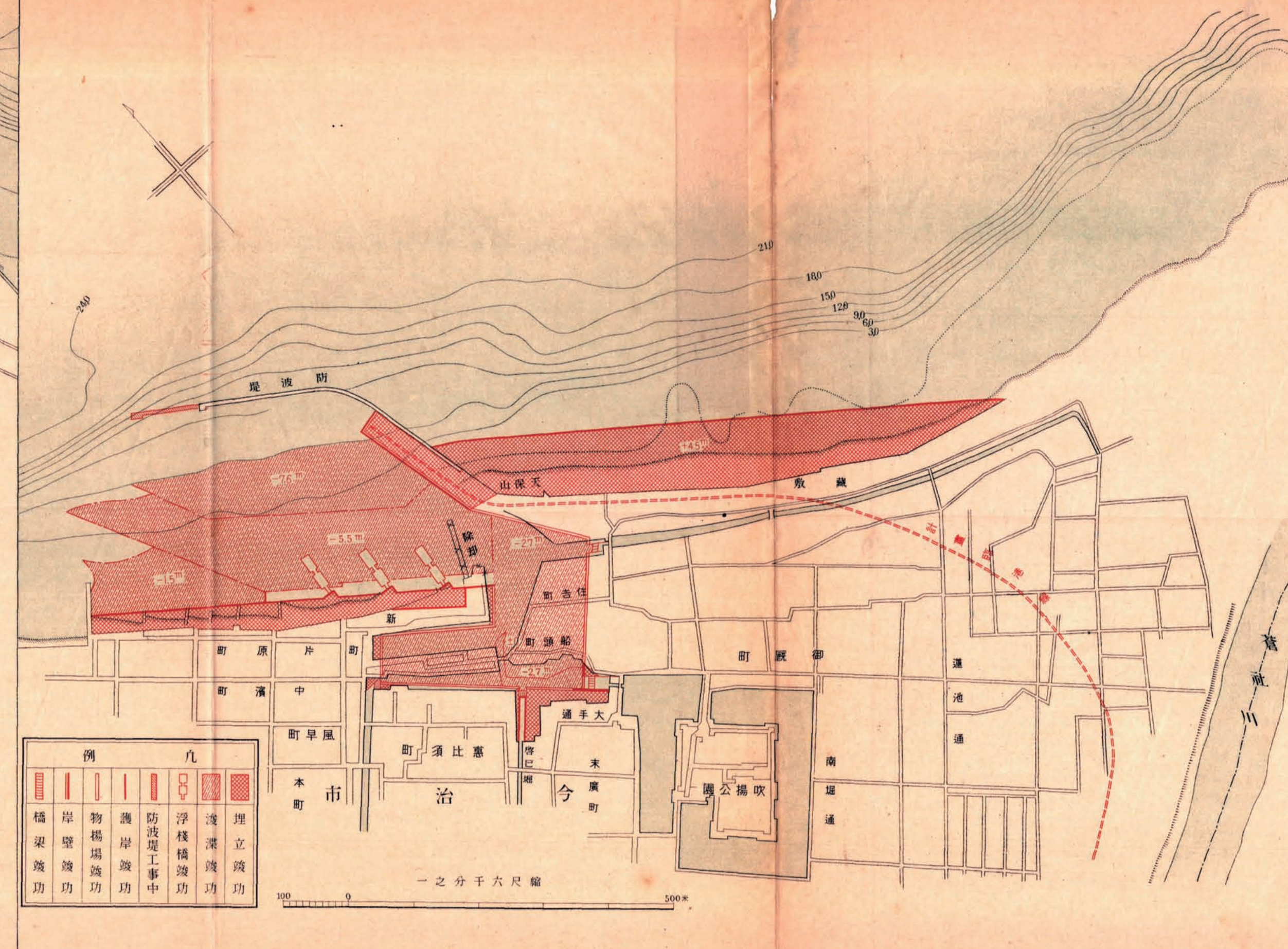
今治港修築工事竣功平面圖
