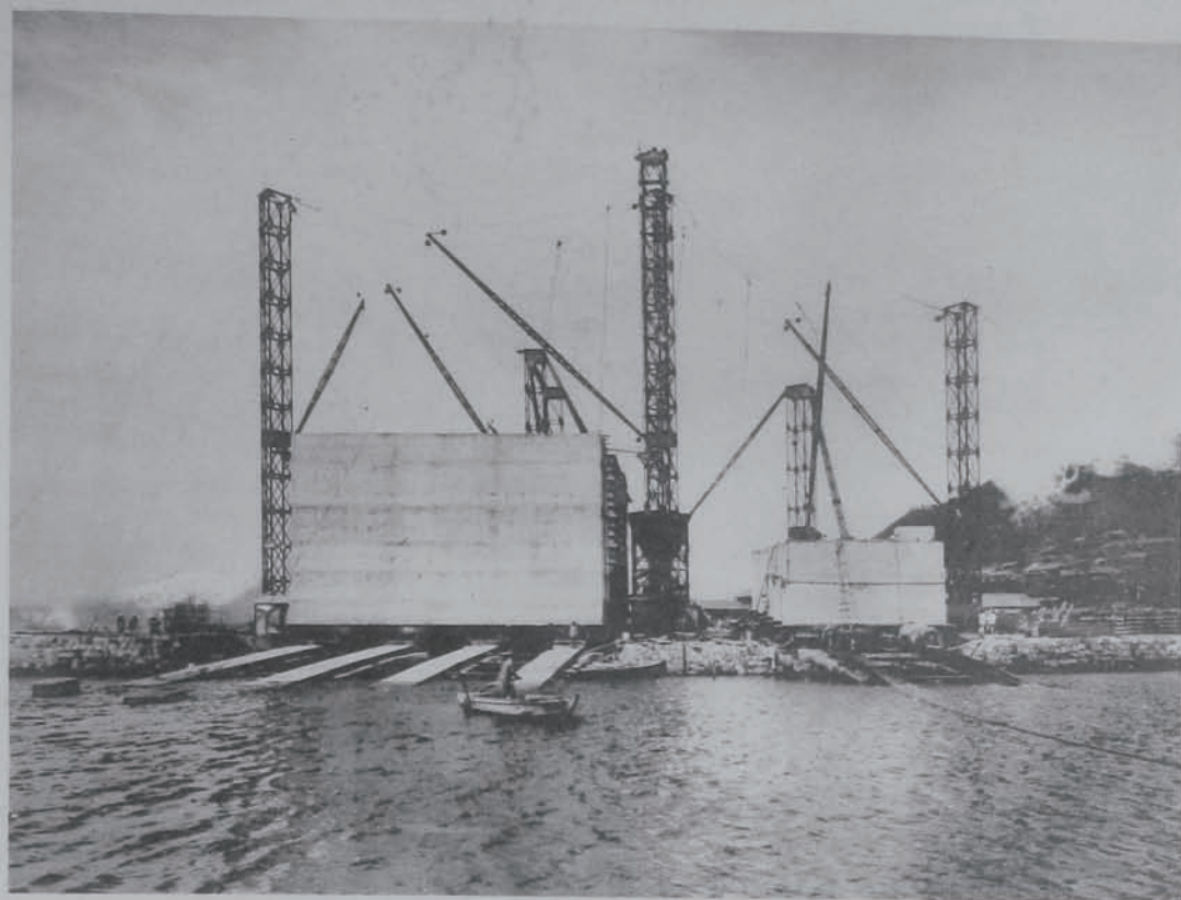
門司港修築工事進水臺上ノケーソ 大重 噸四一・二 尺三六長・尺九三高・六尺九一幅上・八尺二幅下 小重 噸三三・一 尺〇三長・尺六一高・四尺〇一幅上・三尺一幅下 (門司港)
