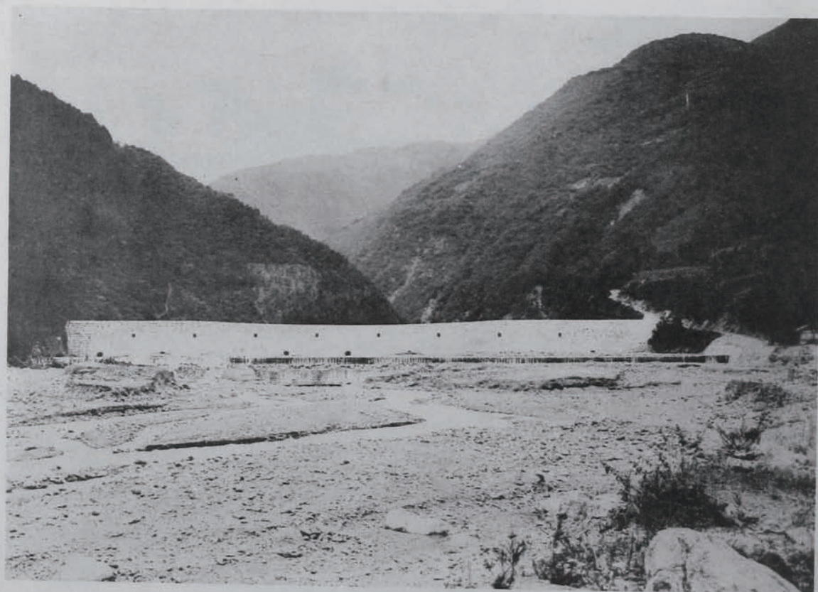
源 堰 堤 竣 功 圖 ( 富 士 川 流 域 御 勅 使 川 砂 防 山 梨 縣 中 巨 摩 郡 村 地 先 )
