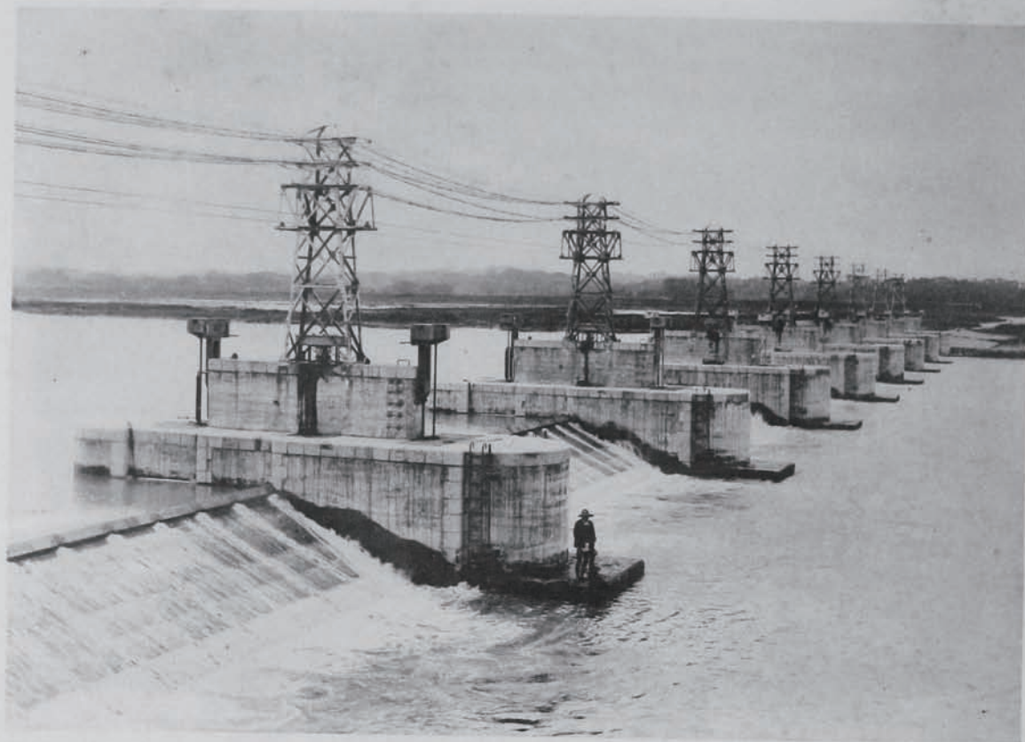
大 河 津 自 在 堰 竣 功 圖 堰 扉 ノ 全 ク 上 リ シ 所 ( 信 濃 川 改 修 新 潟 縣 三 島 郡 大 河 津 村 地 先 )
