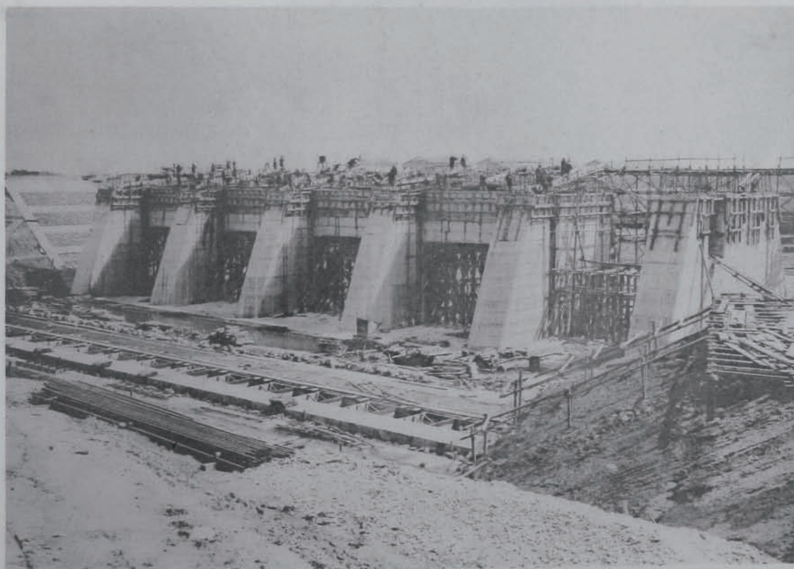
況狀ノ中事工門水節調淵岩 ム望ヲ流下リヨ流上 (先地町淵岩郡島豐北府京東流下川荒)
