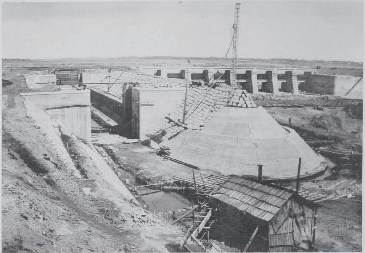
江戶川堰及閘門施工中ノ狀況
