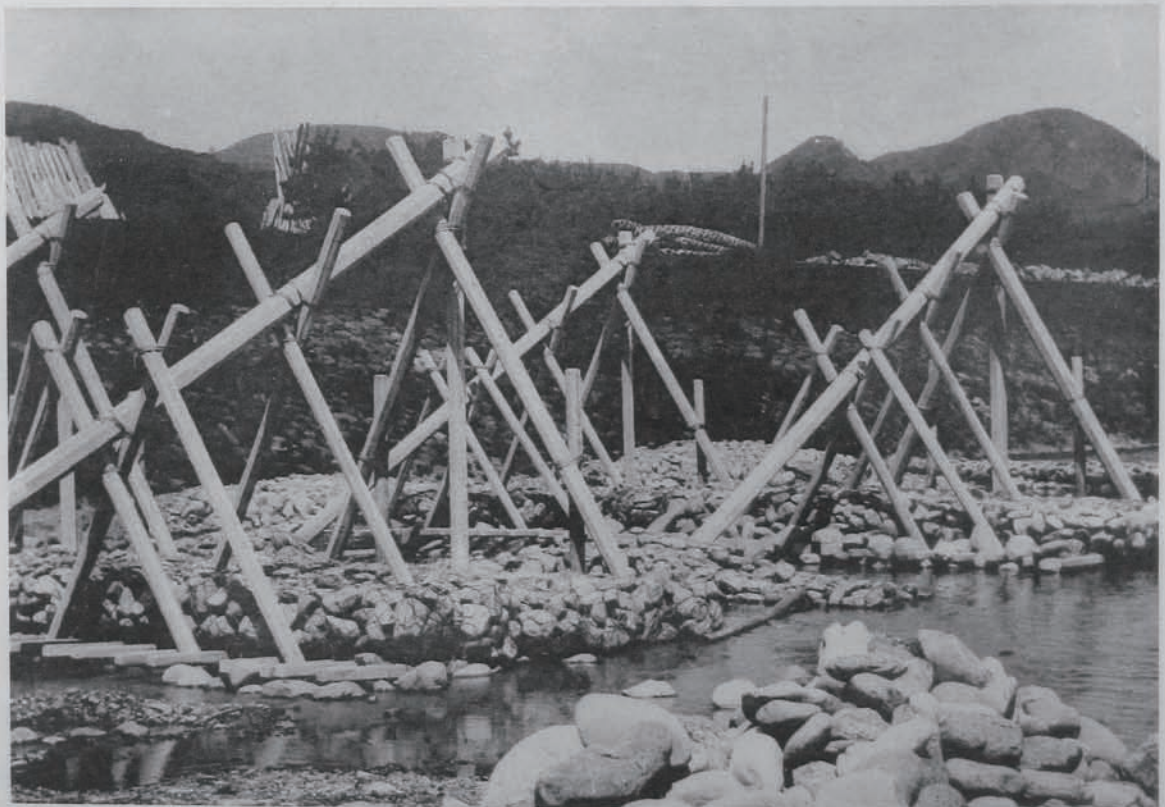
（靜岡縣庵原郡富士川町大字岩淵）中之鄉制水補修後ノ狀況 泥凝土大壩一箇四組宛二箇所設
