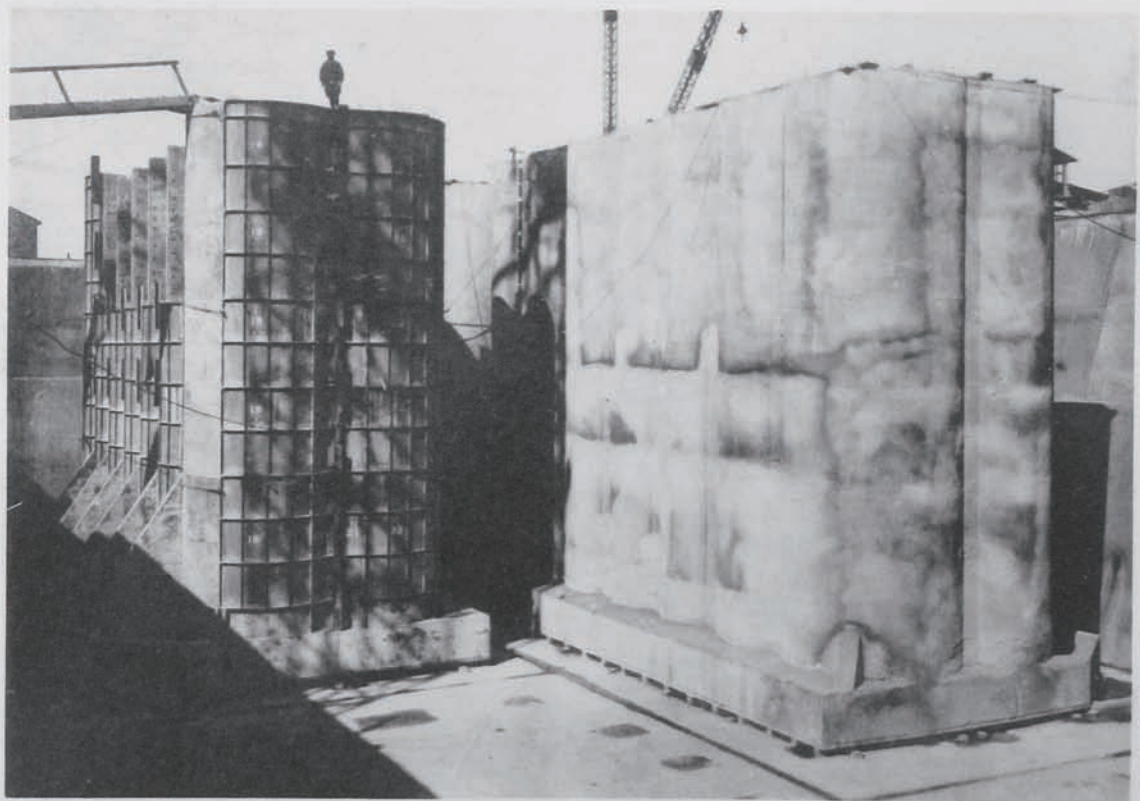
内渠船函造事工築修港濱横
