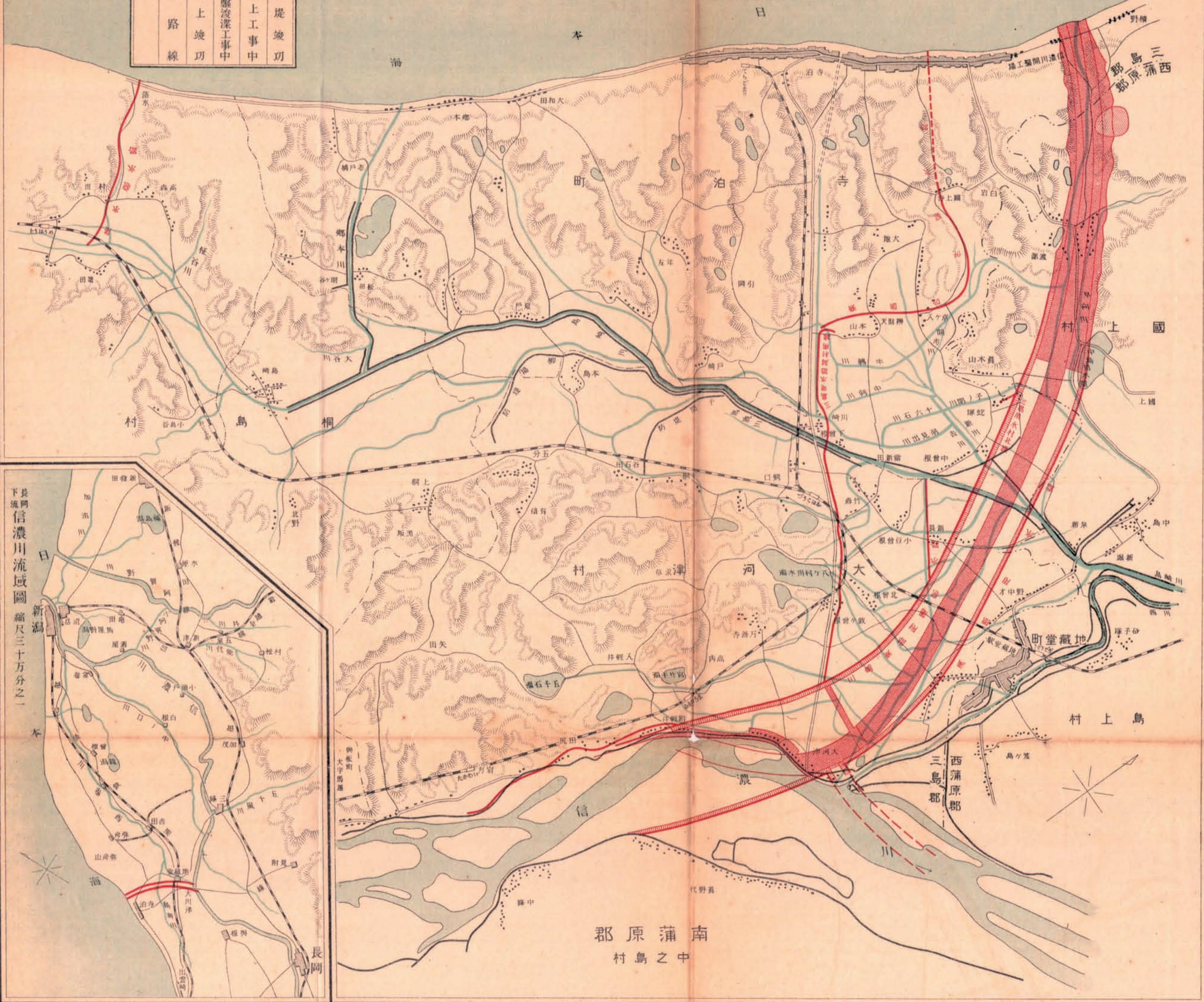
信濃川改河工事平面圖 縮尺一萬八千分之一
