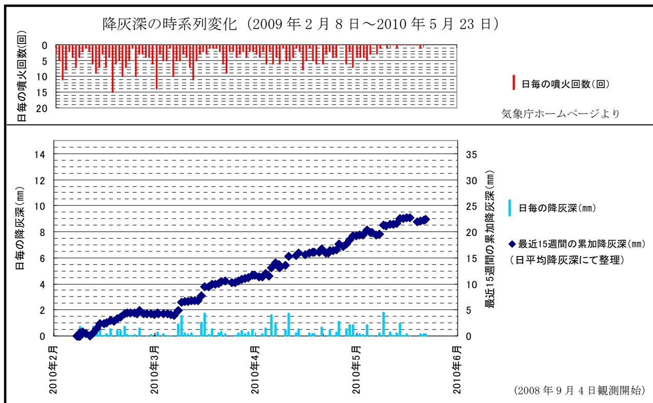
図 2 最近 15 週間の累加降灰深の推移
