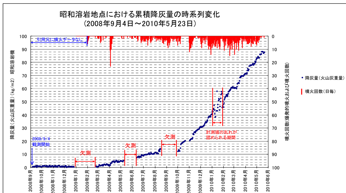
図 3 自動降灰量計による降灰量の推移（2008 年 9 月～2010 年 5 月）
