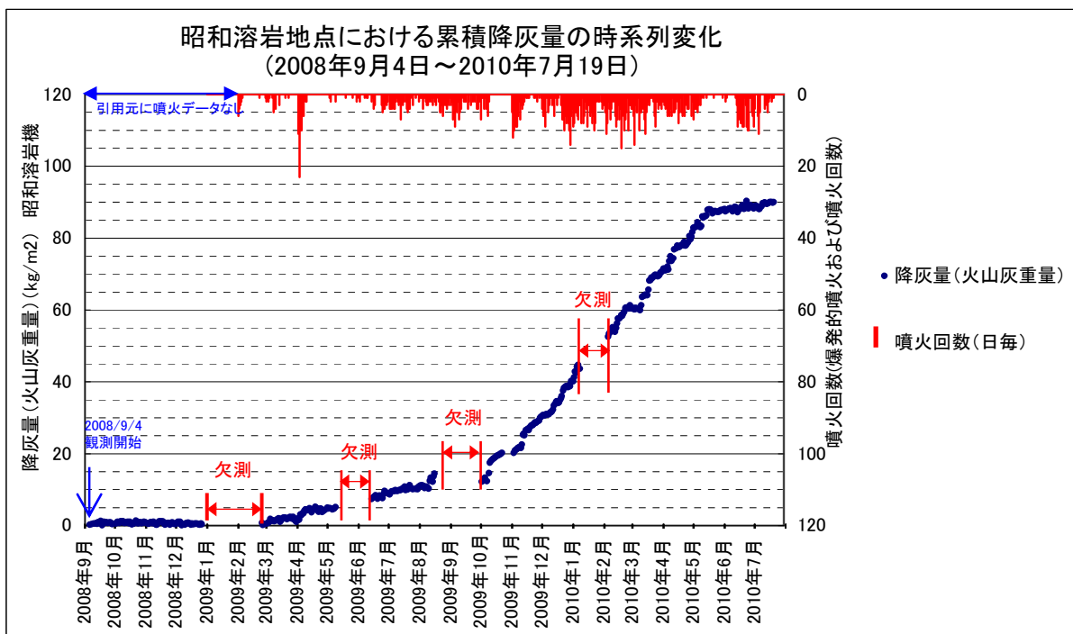
図3 自動降灰量計による降灰量の推移(2008年9月～2010年7月)
