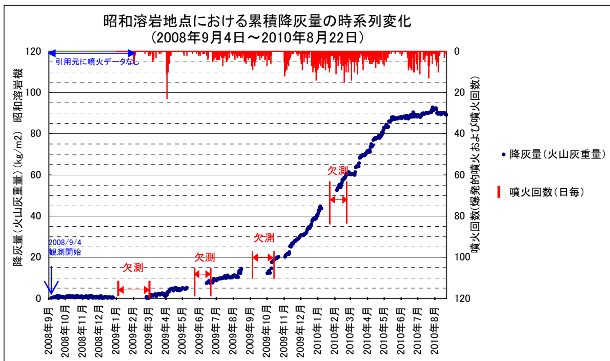
図3 自動降灰量計による降灰量の推移(2008年9月～2010年8月)
