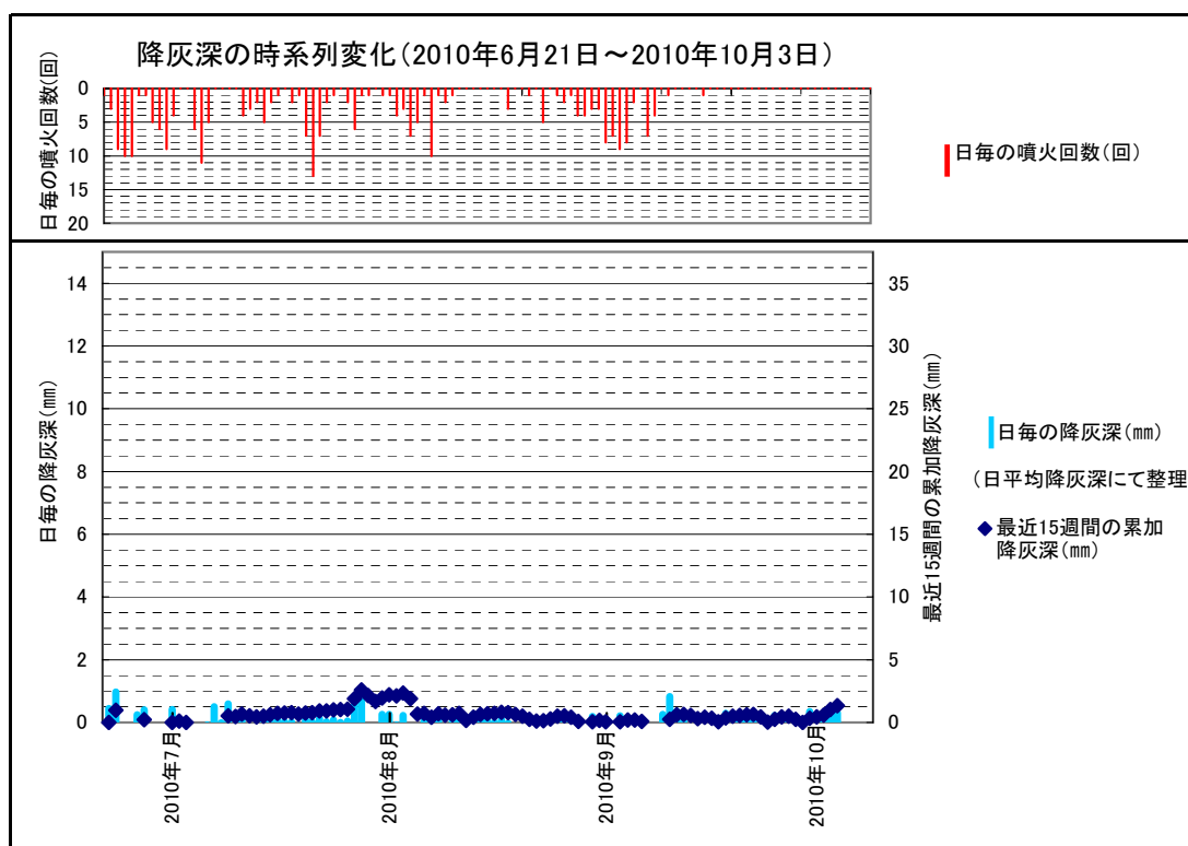
図2 最近15週間の累加降灰深の推移
