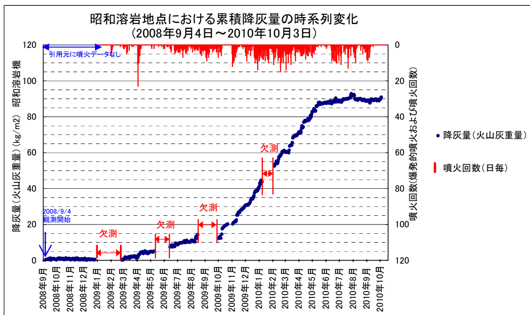
図3 自動降灰量計による降灰量の推移(2008年9月～2010年10月)
